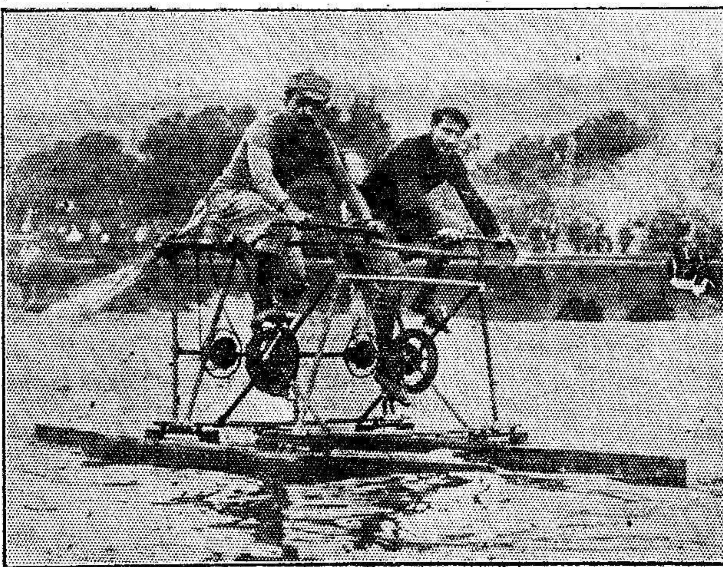
Hidrocielo con hélices aéreas de los hermanos Moretti, que ha sido ensayado con excelentes resultados en Napoles.
