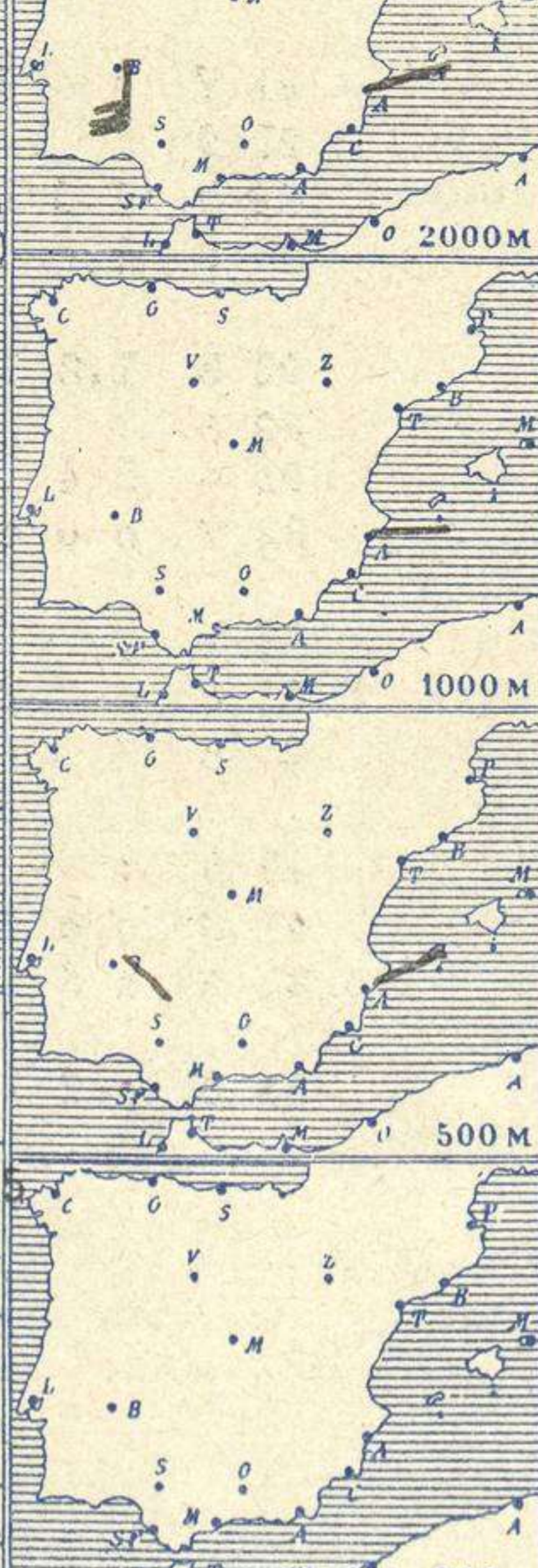
Observaciones en Madrid de 13 h del día 13 a 7 h del día 14
