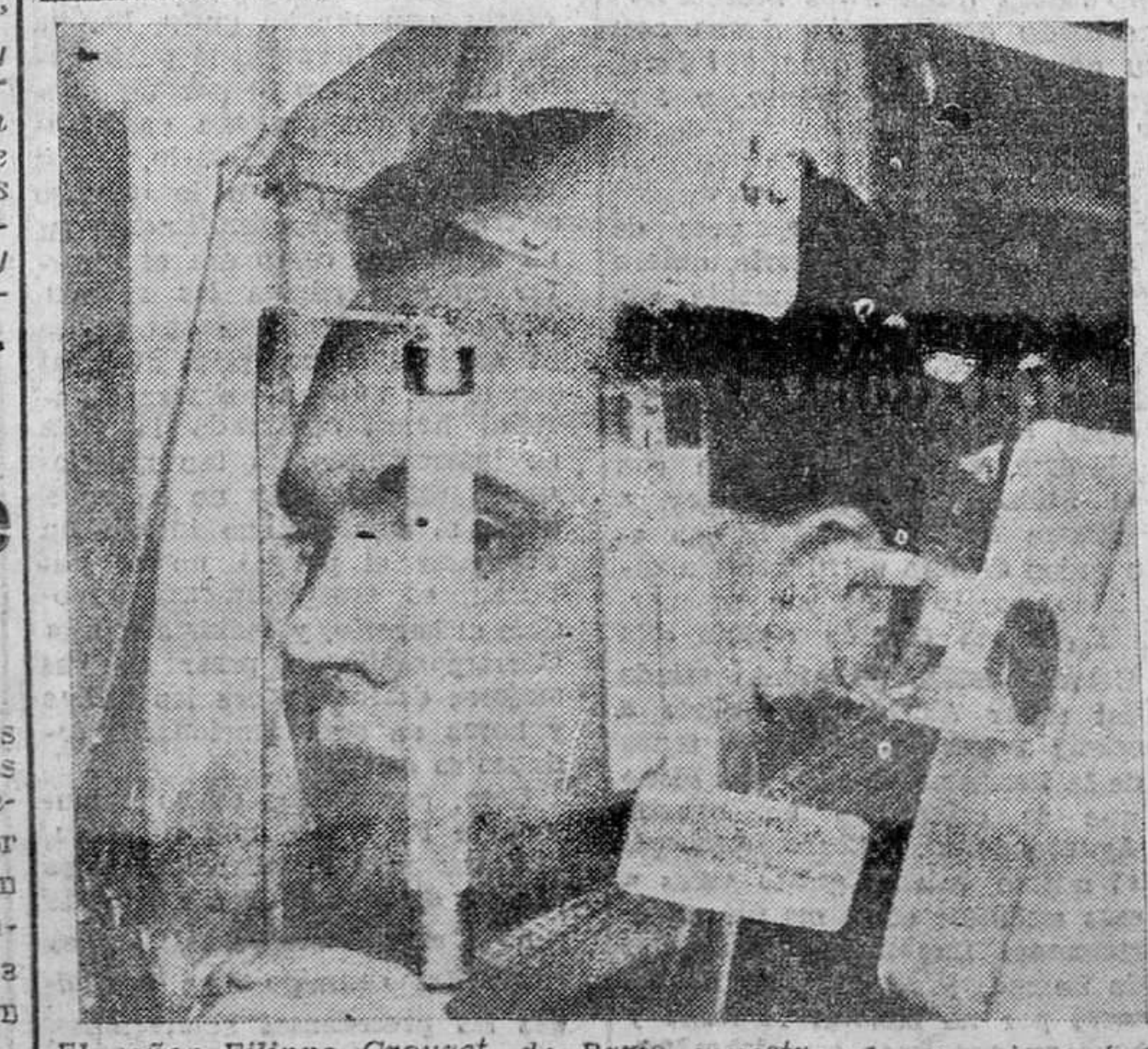
El señor Filippo Crouzet, de Paris, muestra el caso inventado por él destinado a los motoristas irioleros. Consiste de un recipiente herméticamente cerrado de materia plástica, el cual lleva dentro un tubo generador de aire corriente que le proporciona una temperatura de cinco grados en el exterior y veinticuatro en el interior. Lo que se llama calefacción motorista.
