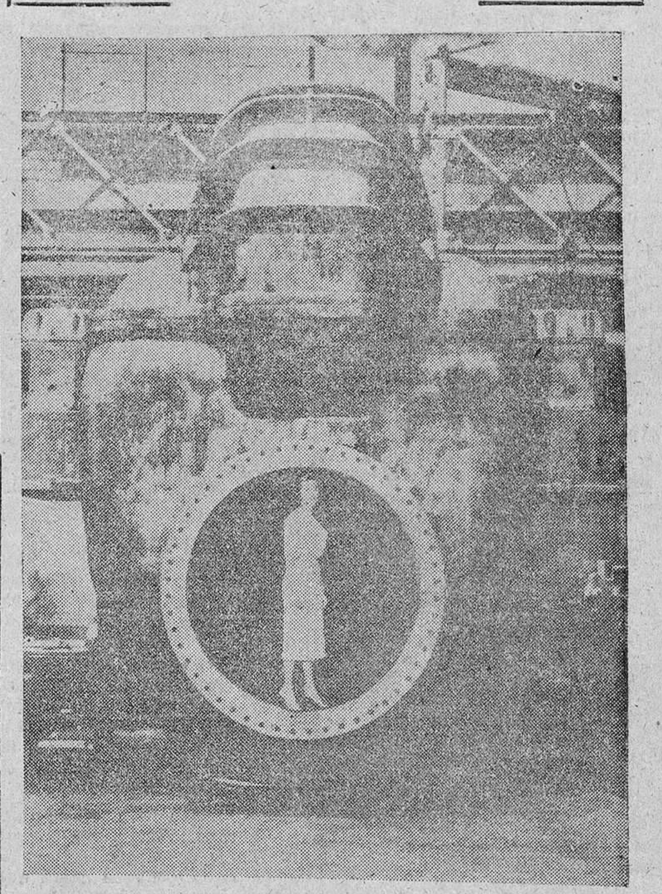
La mayor bomba de cuantas se han fabricado hasta la fecha en el mundo, con un peso de ochenta toneladas, acaba de ser terminada en la factoria de Worthington de Harrison (Nueva Jersey). Está destinada al servicio de los alcantarillados de Río de Janeiro, y tiene una capacidad de un millón de litros por minuto.
