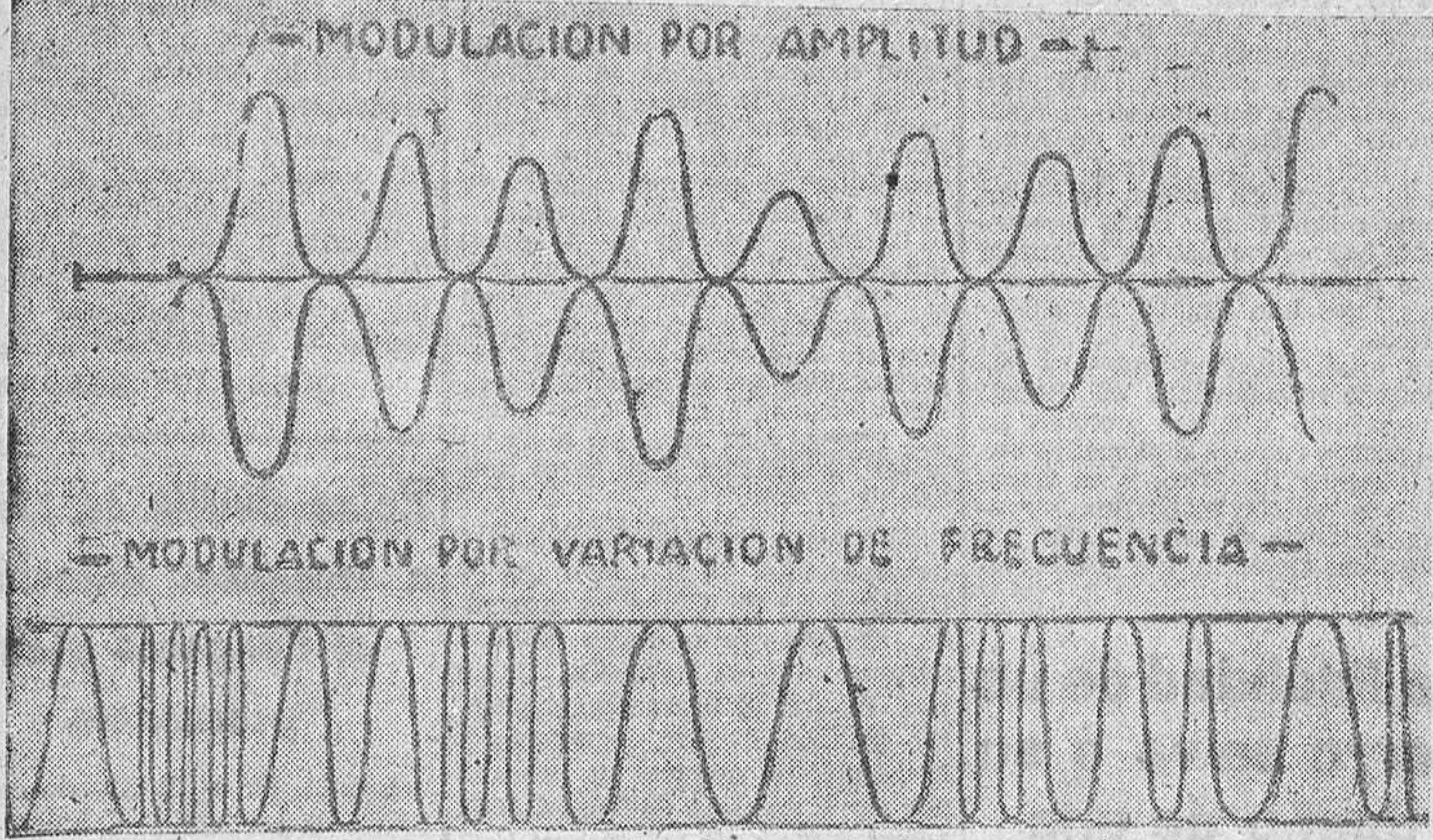
Estos dos gráficos muestran la diferencia que existe entre la onda portadora con que radian las emisoras locales actualmente y la señal de frecuencia modulada que va a ser instalada dentro de poco en toda España.
