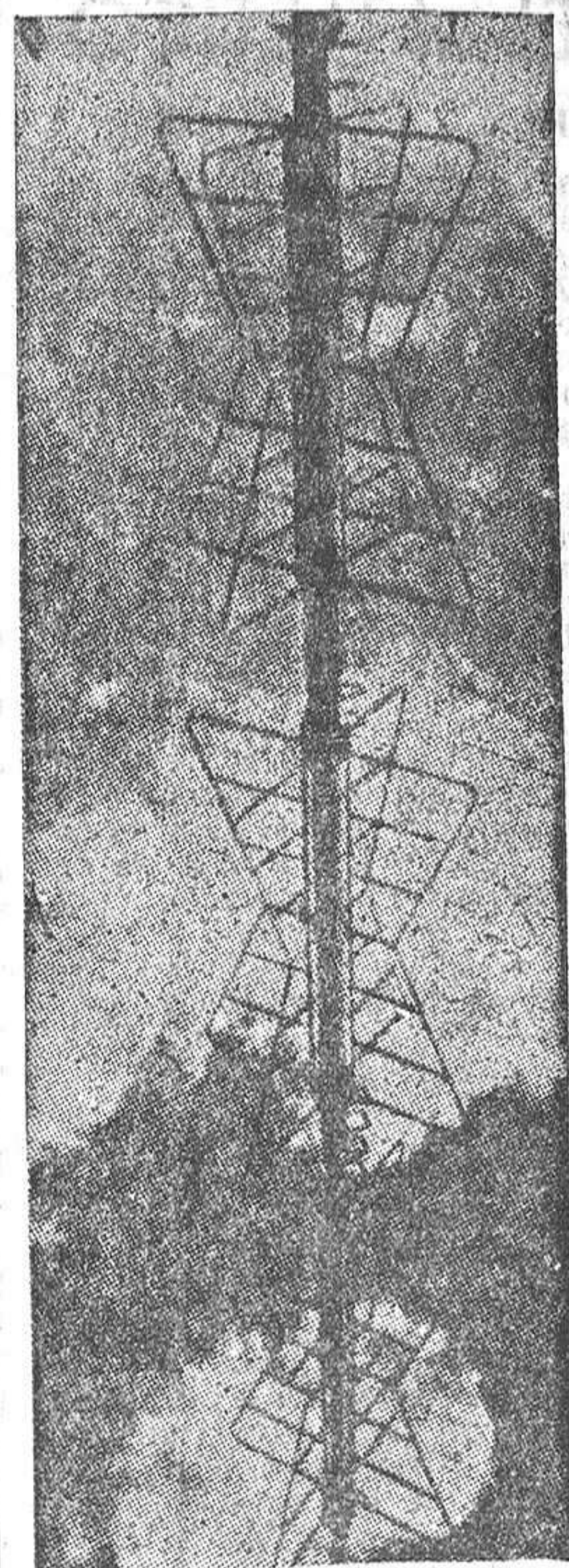
Sistema de antena de televisión «superturstile», de tres elementos, instalada en Chamartín.
