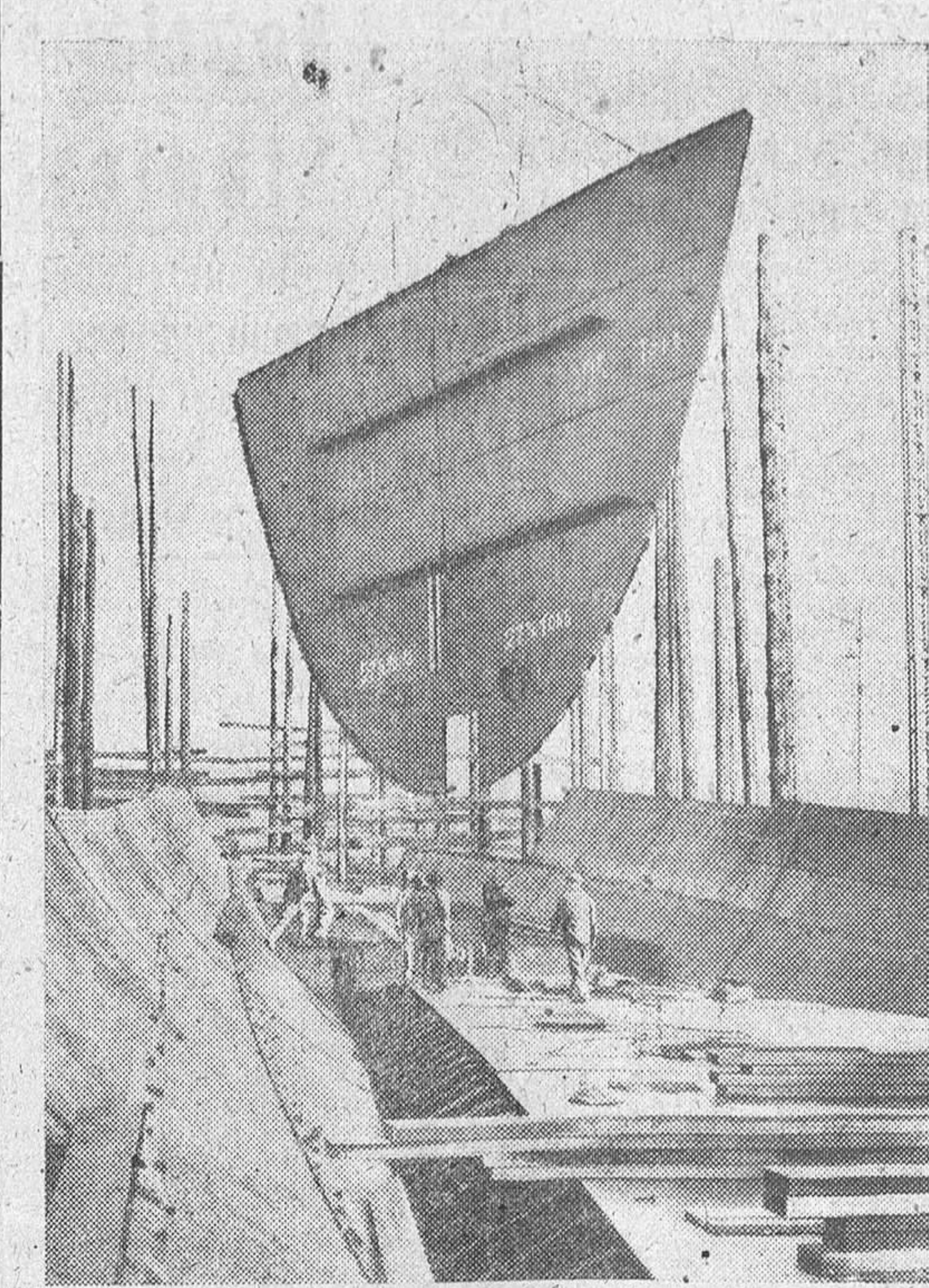
En enero del presente año se emplearon por vez primera, piezas de buques prefabricadas, en la construcción del «ORCADES». Este nuevo método significa un ahorro de 900 toneladas de acero en la construcción de buques de esta clase; un aumento en la capacidad de carga hasta 2.000 toneladas aproximadamente; reduce la vibración y, además, ahorra un 25 por 100 de tiempo en la construcción de los mismos.
