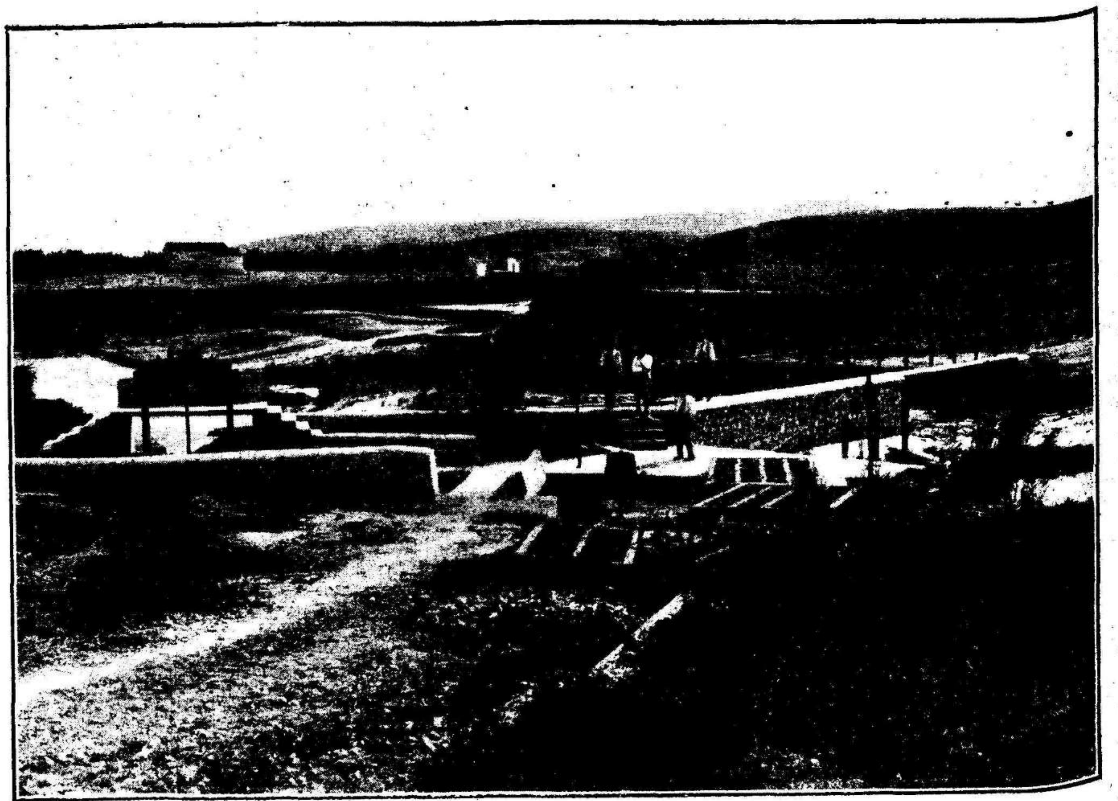
VISTA GENERAL DE LA CONTRAPARADA. — Al fondo la Presa; a la derecha el muro de contención de la C.A. de Compuertas para los desagües y a la izquierda el primer tablao de la acequia mayor de Aljufía.
