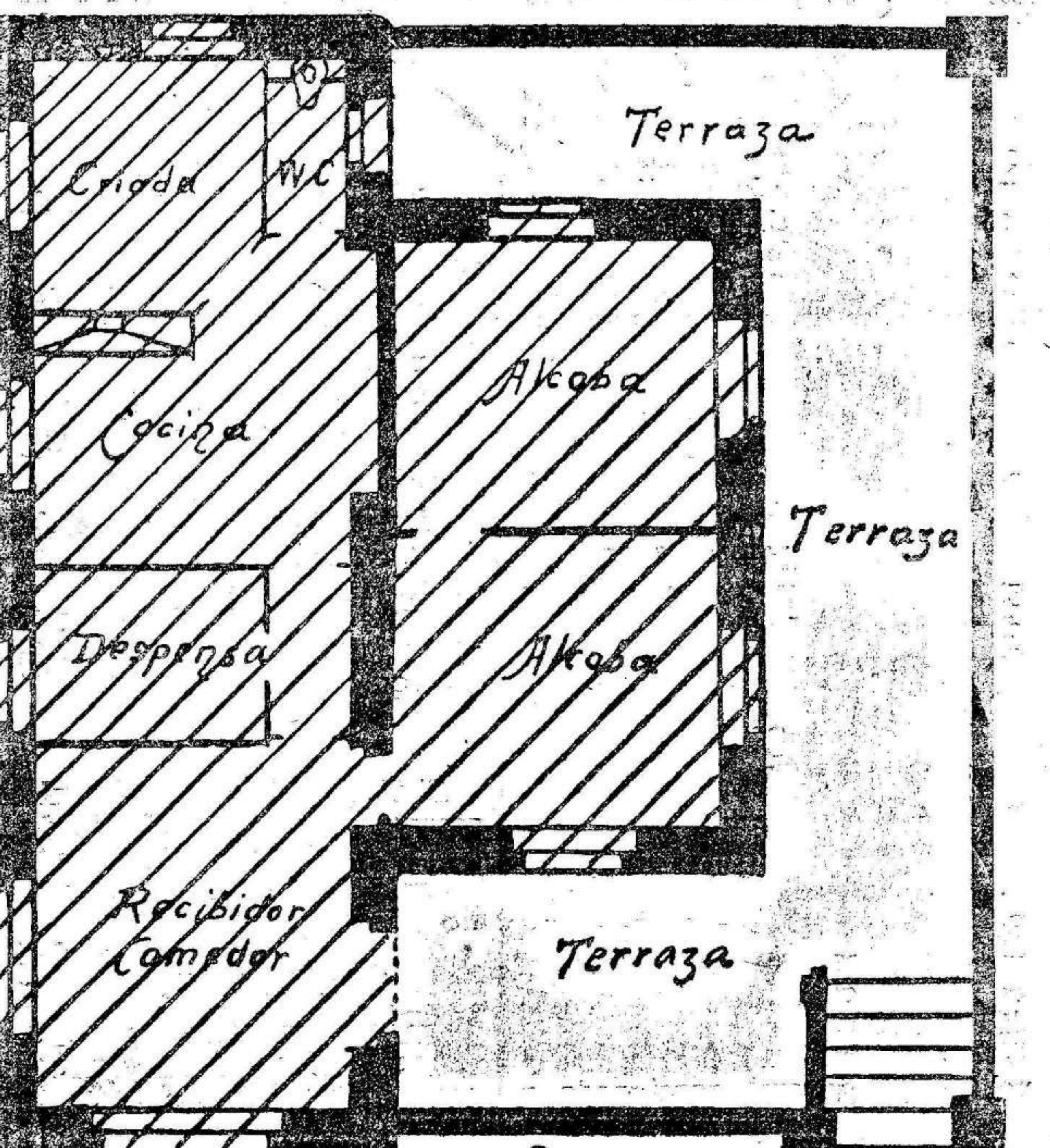
Plano de la casa-hotel, regalo de EL LIBERAL.
