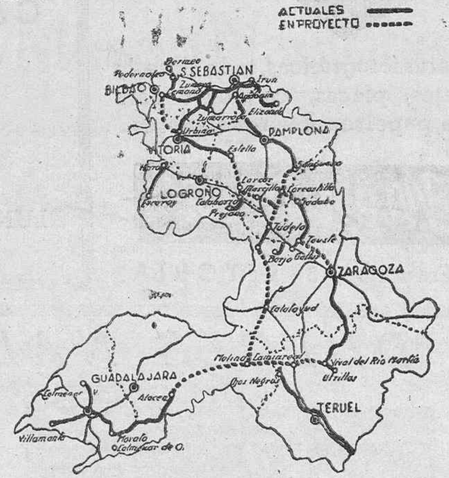
FERROCARRILES DE VIA DE UN METRO
