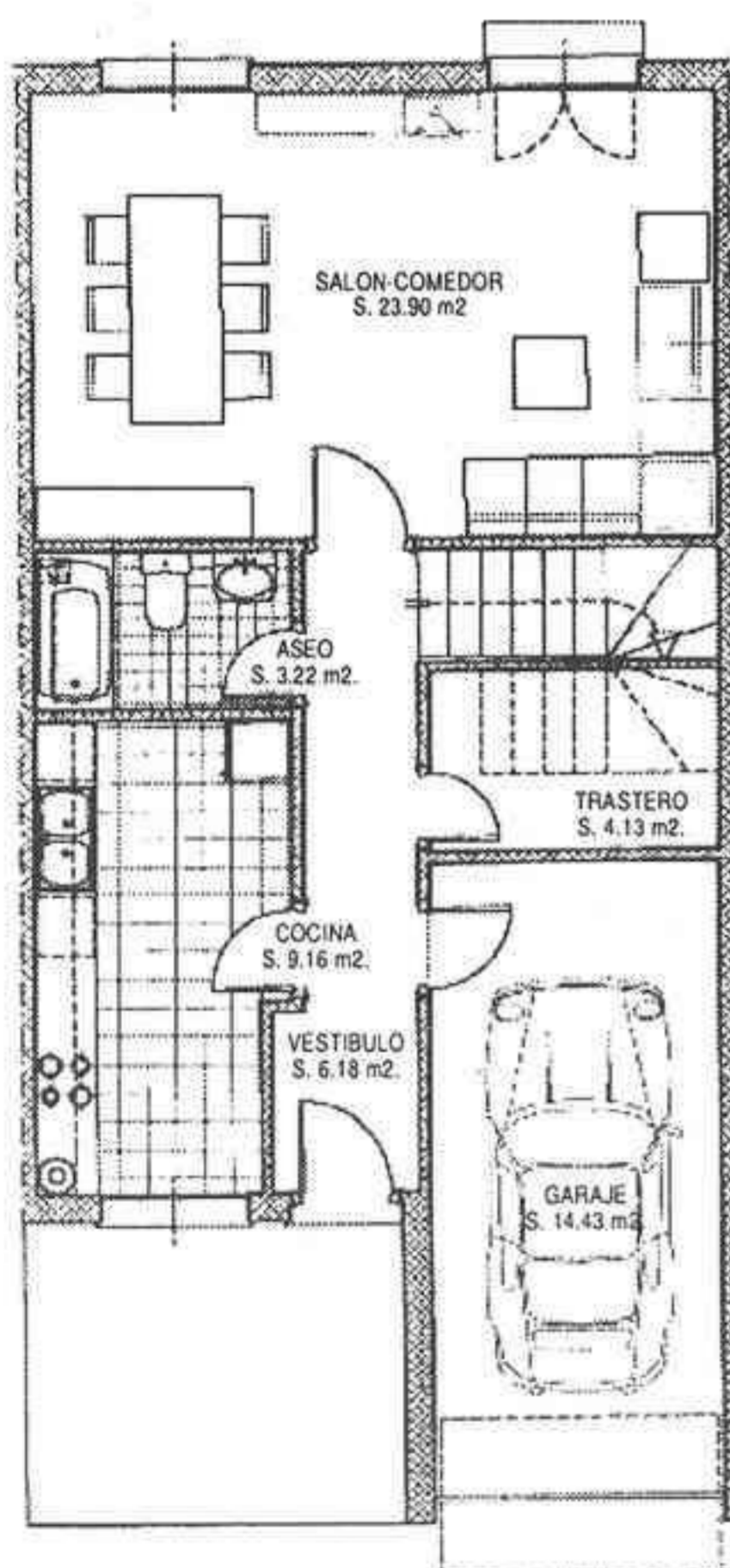
PLANTA BAJA
