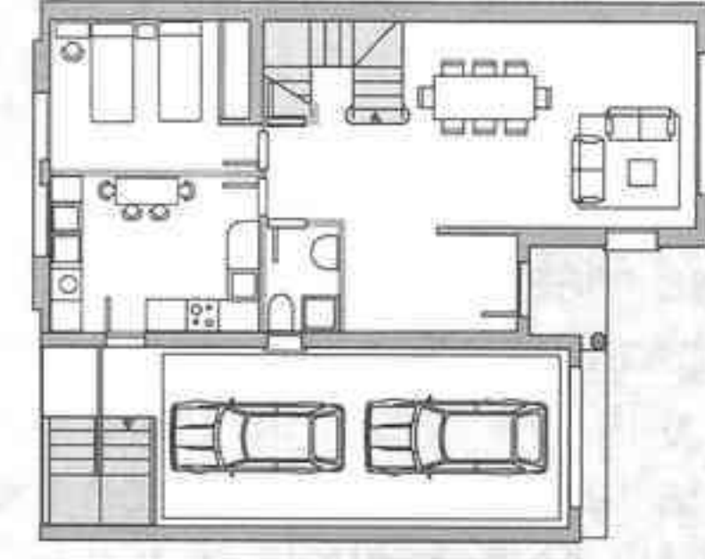
Modelo Herrera Individual, 4 dormitorios Sup. construida 232,82 m 2
