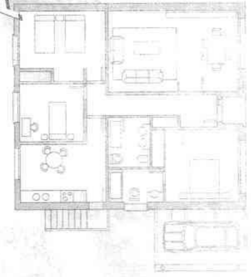
Modelo Villanueva Individual, 3 dormitorios Sup. construida 108,10 m 2
