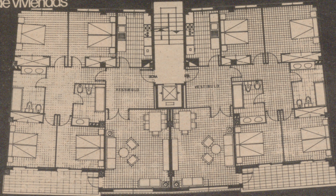
Plano de viviendas
