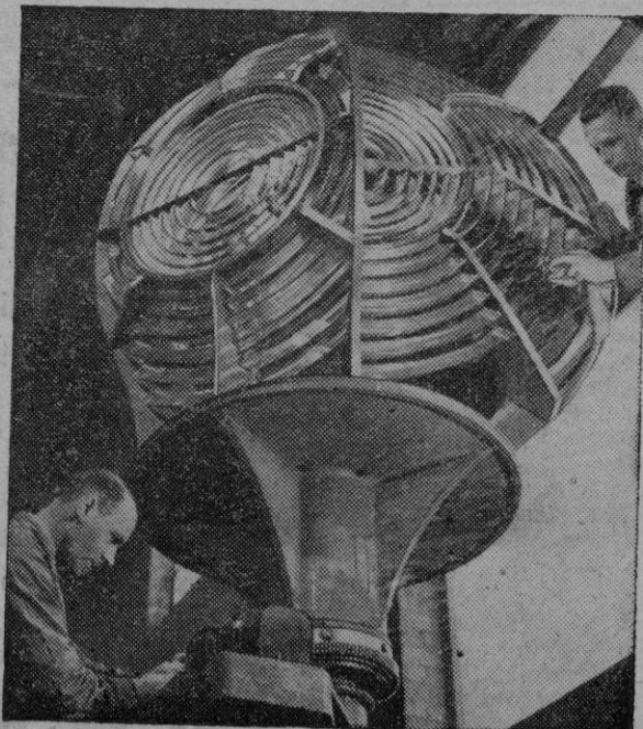
El sistema óptico construido para el faro de Ytteroeerne, en Noruega, será uno de los más potentes del mundo; pesa dos toneladas y será montado sobre una columna de 6'10 metros de alto
