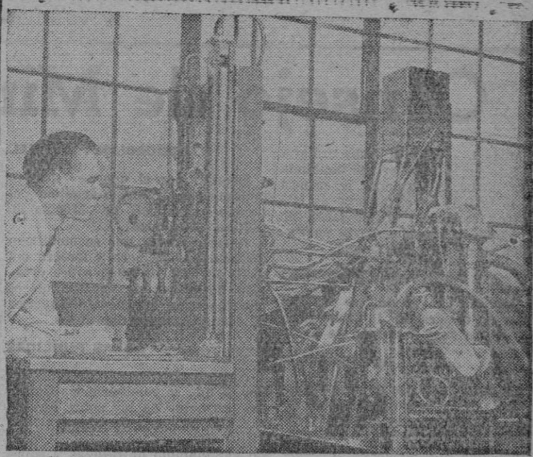
Investigaciones Industriales en la Gran Bretaña. — Pruebas efectuadas sobre un motor de un cilindro para observar el funcionamiento de sus partes. Los instrumentos de control en el panel, indican la velocidad, consumición de gasolina, y la temperatura concentrada en varias partes del motor propiamente dicho.
