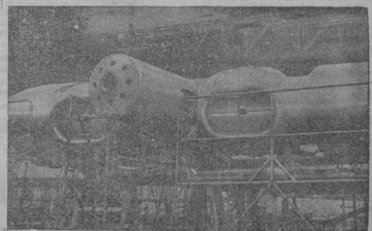
Uno de los últimos tipos de avión que se están construyendo en Inglaterra es el soberbio «Bristol Brabazon I». Su radio de acción es de 8.000 kms. Lleva 8 motores de propulsión a chorro de gas. Tiene capacidad para 80 pasajeros y dispone de camas para todos ellos
