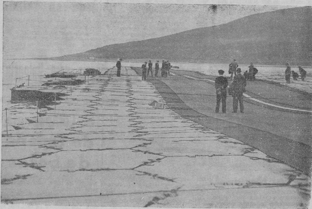
He aquí una foto de «Lily» la primera isla flotante del mundo, construida por ingenieros británicos bajo la dirección de su inventor Mr. R. A. Hamilton.
