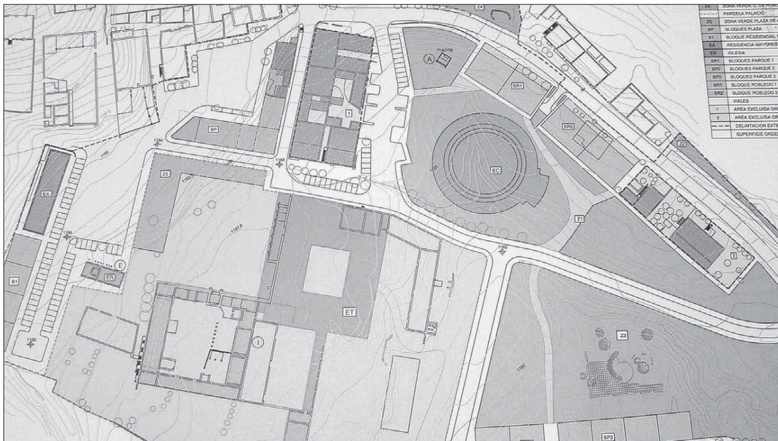
Plano del proyecto previsto de rehabilitación y recuperación del Palacio de Valsain y su entorno. /EL ADELANTADO
