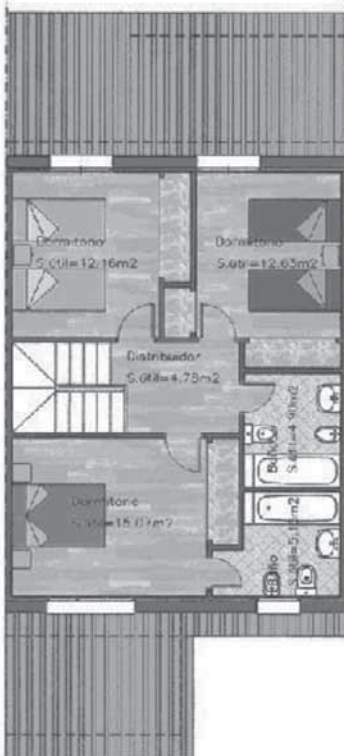
Planta alta S.const.=68,60m 2
