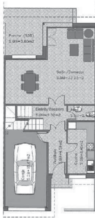
Planta baja S.const.=93,08m 2
