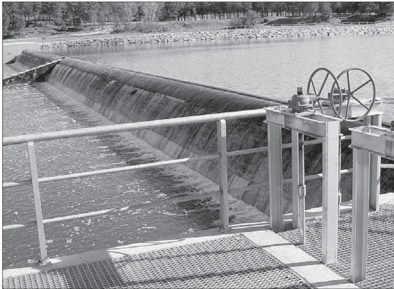
Minipresa hecha en Aldeanueva del Codonal para la acumulación de agua del arroyo Barrascas PENALOSA
