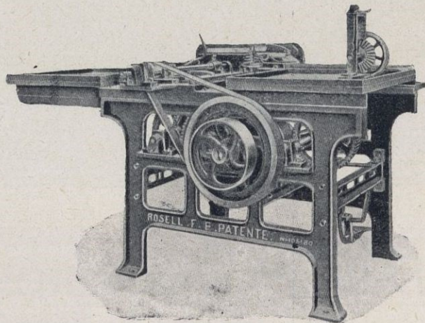
Nueva máquina para coser suelas de alpargata Construcción Nacional Patente núm. 105180
