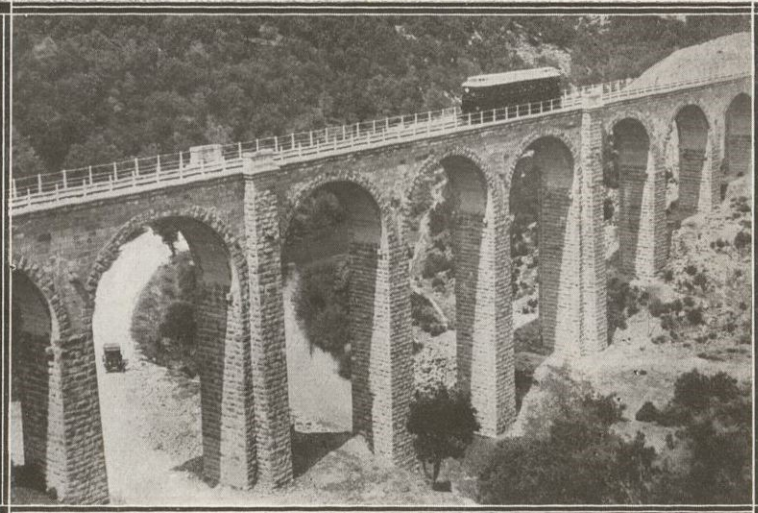
Navarra: Uno de los magníficos puentes construídos para el nuevo ferrocarril Vitoria-Estella, inaugurado por el Presidente del Consejo señor Primo de Rivera durante su reciente estancia en Vitoria
