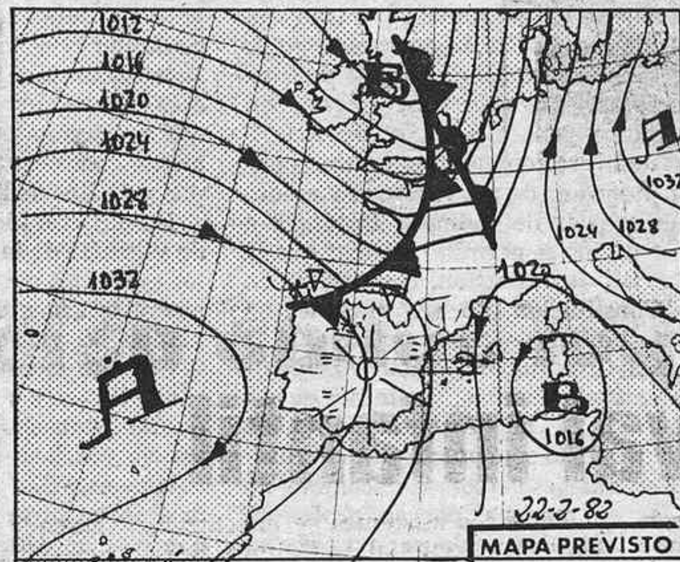
Situación anticiclónica sobre el país, con frentes nubosos rozando las costas septentrionales peninsulares
