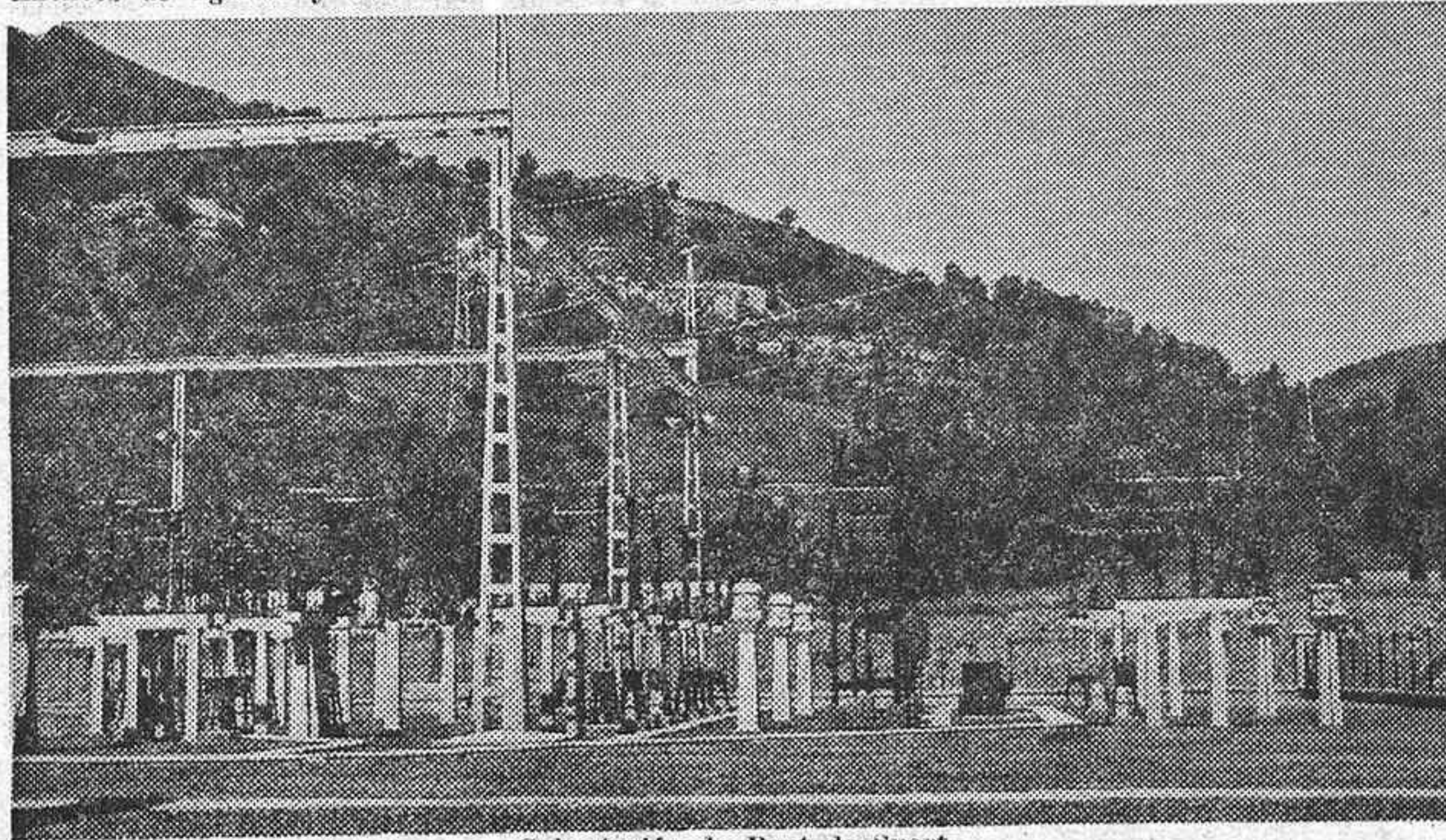
Subestación de Pont de Suert
