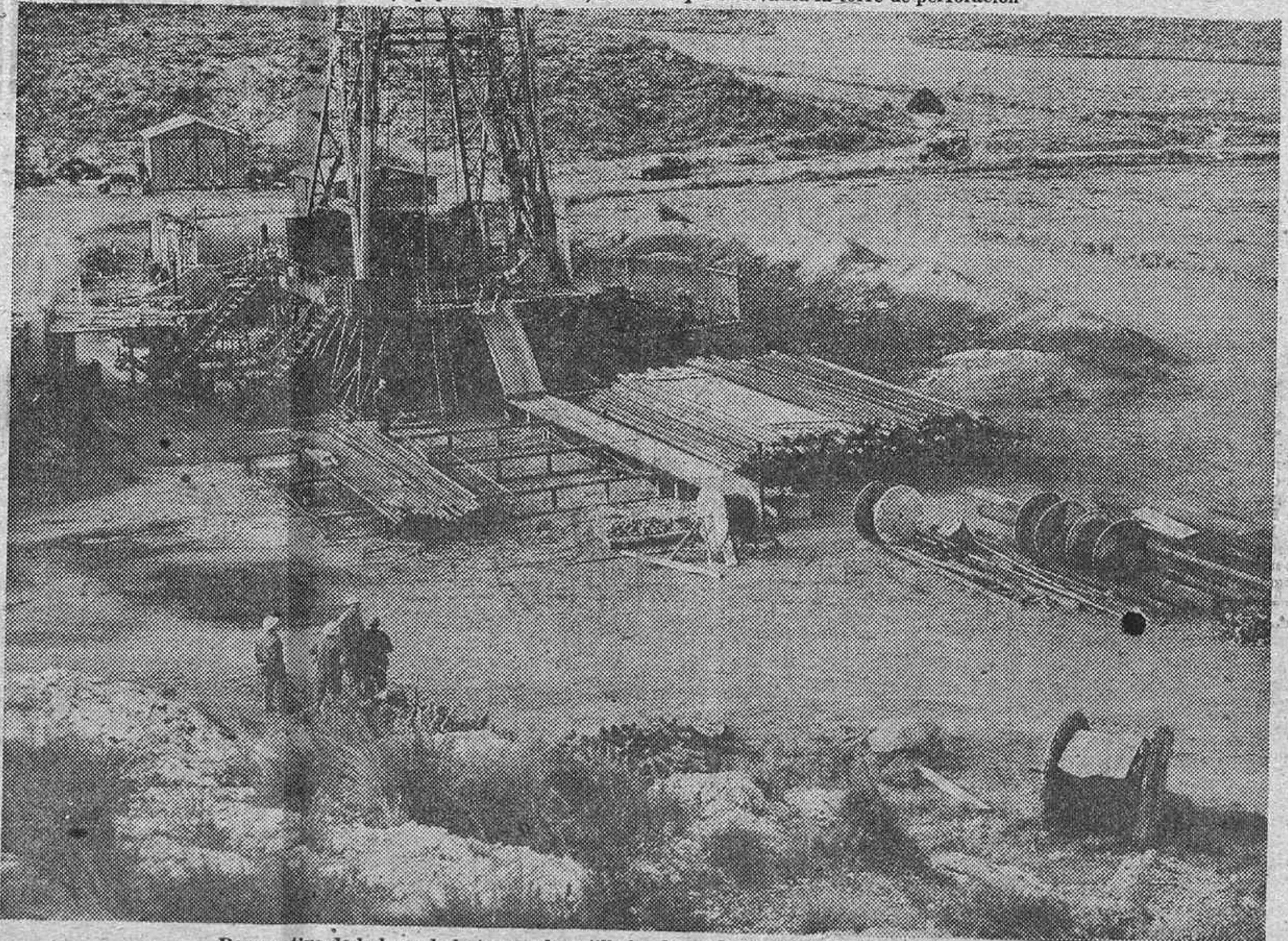
Perspectiva de la base de la torre y los utilajes de sondeo en las cercanías de Gelsa de Ebro
