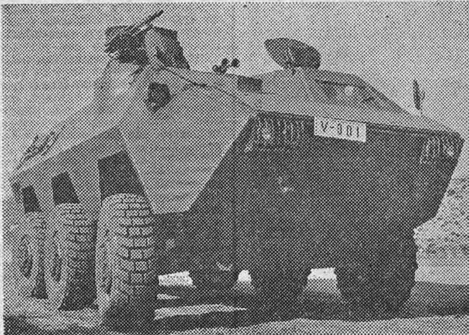
BMR-600, con motor de 352 CV., suspensión independiente a cada rueda, frenos de disco, dirección a ejes extremos y capaz de navegar a 8 km/hora
