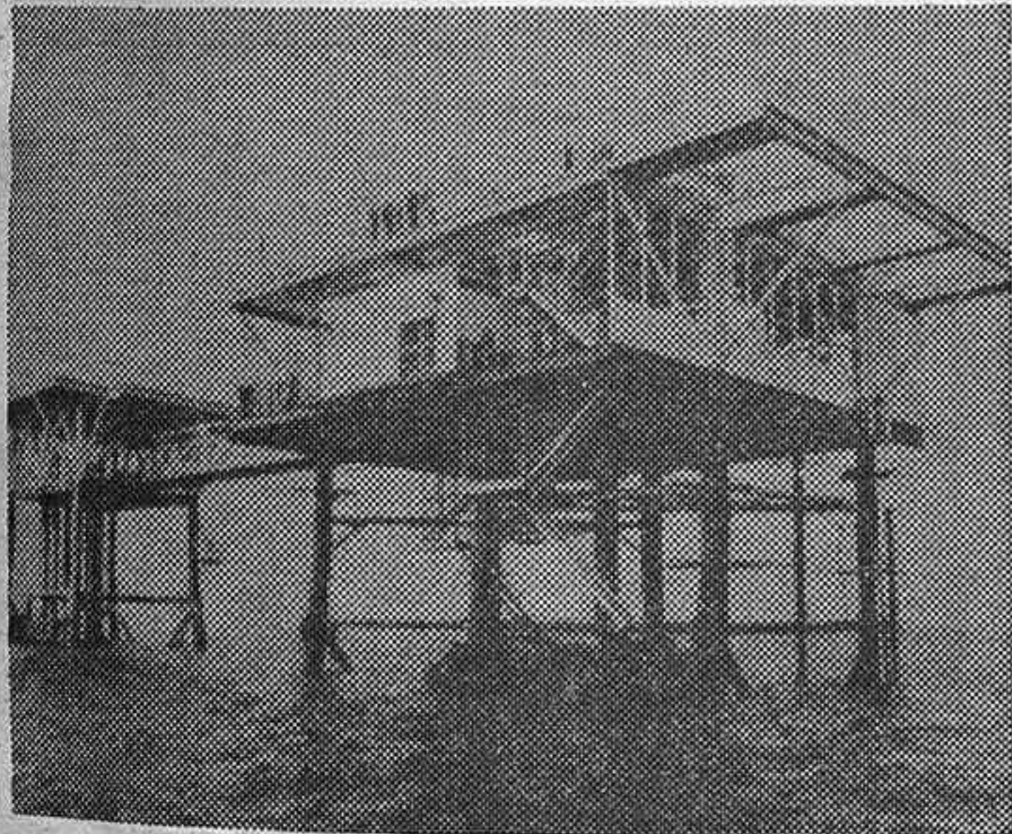
Plataforma de producción en Amposta
