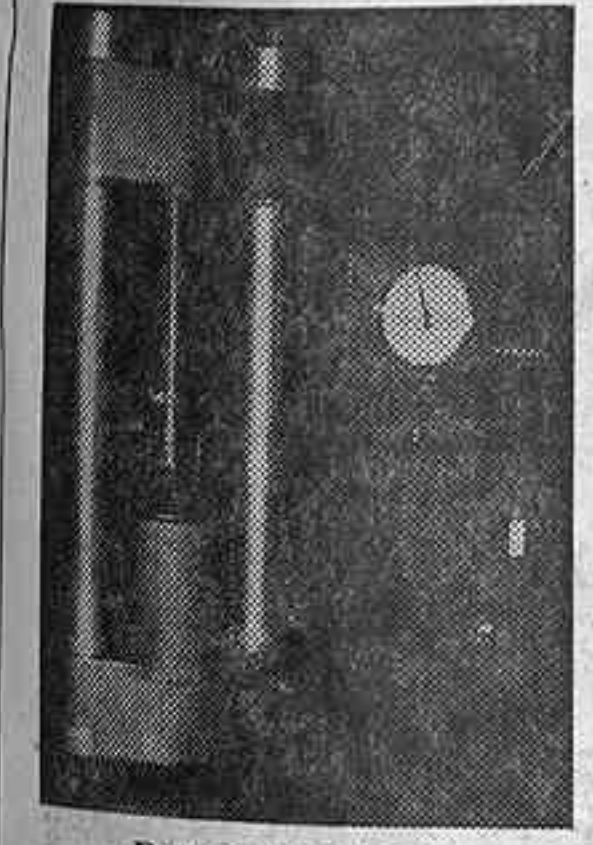
Prensa hidráulica para ensayo de hormigones de hasta 300 toneladas
