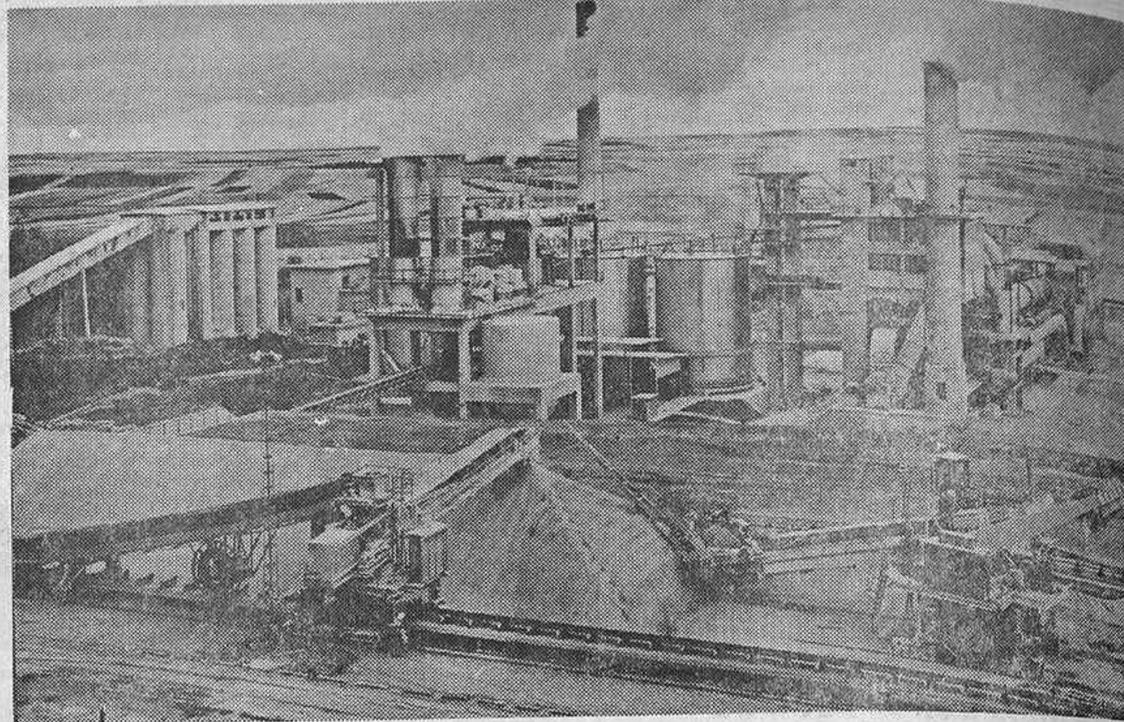
Moderna instalación de prehomogeneización de materias primas de FIVES LILLE-CAIL IBERICA en una fábrica de cemento de Villaluenga de la Sagra (Toledo)
