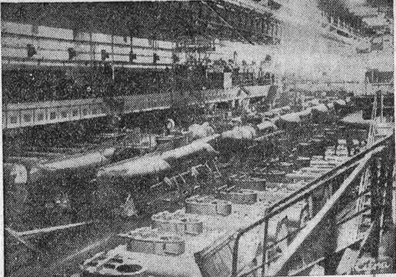
En las antiguas bases navales alemanas, y más especialmente en la de Wilhelmshaven, han sido encontrados gran número de submarinos en proceso de construcción o listos para su entrega a la flota. He aquí un taller de la citada base de Wilhelmshaven, donde se hallaban a punto de ser terminados numerosos submarinos enanos con capacidad para dos tripulantes. (Foto Cifra.)
