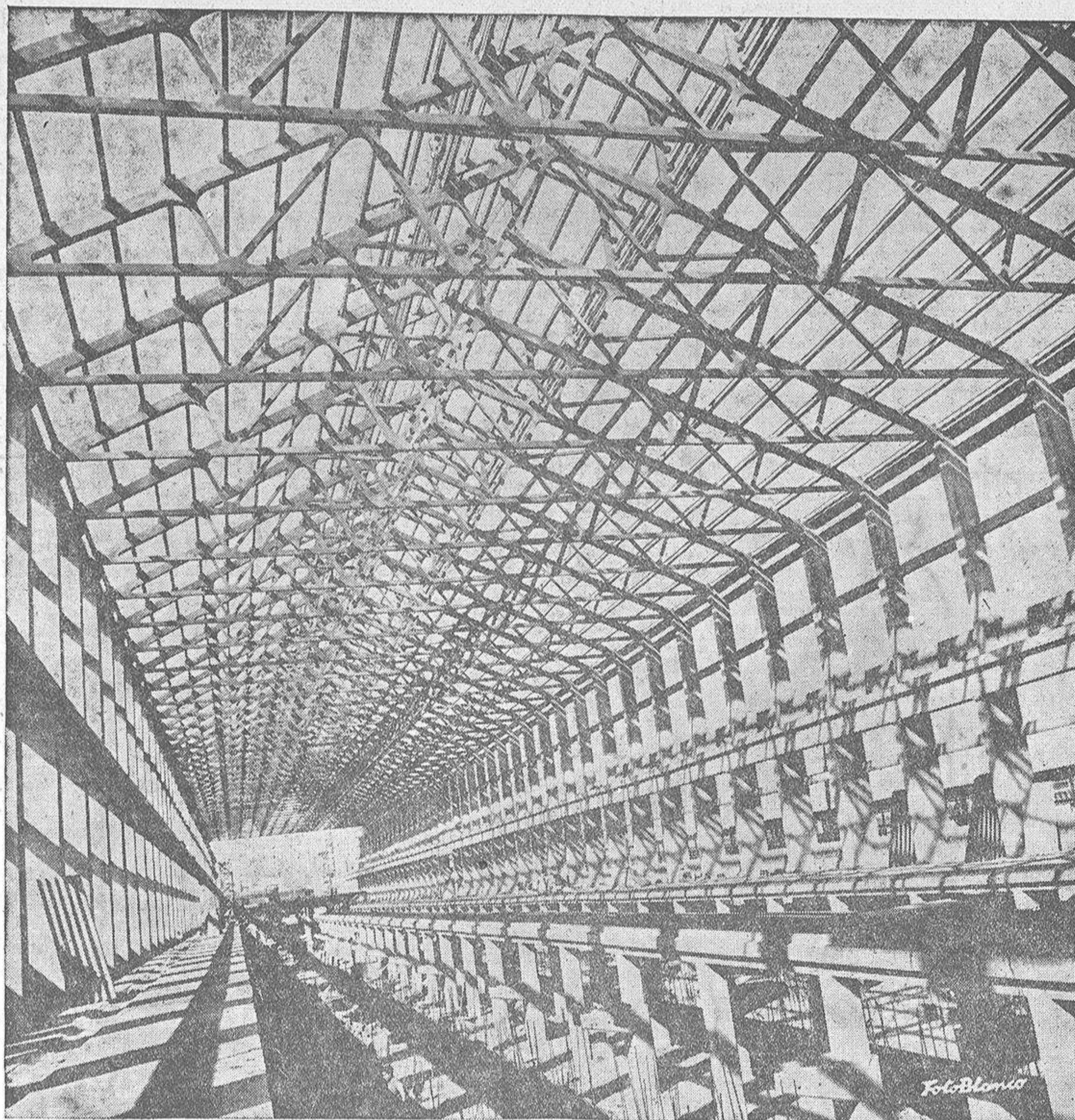
Nave de 25 mts. de luz, con cerchas a 5 mts., para Fibrocemento en ALUMINIOS DE GALICIA, S. A., de La Coruña (Zona industrial de la Grela).
