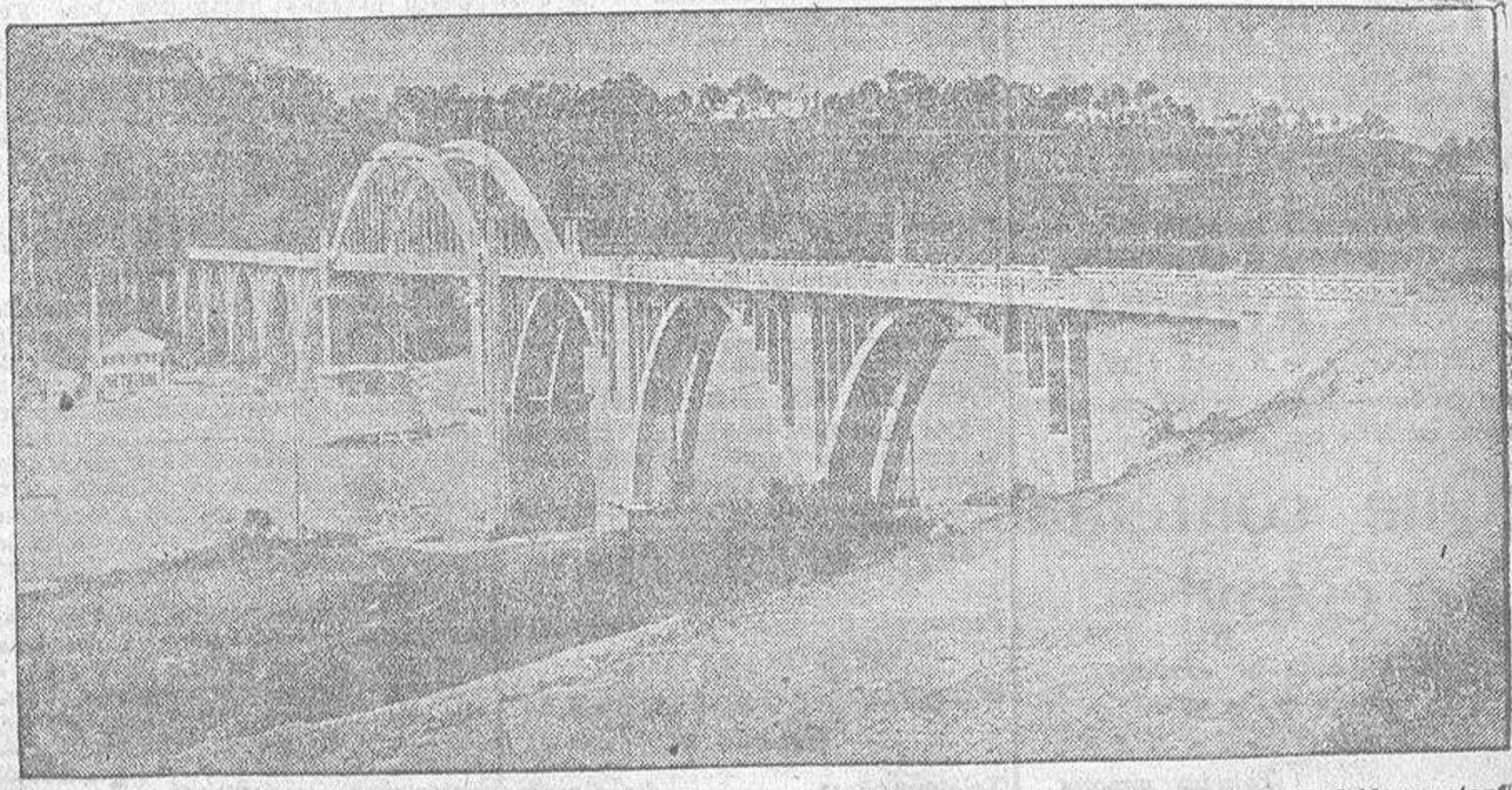
Otra gran obra iniciada hace muchos años y que va a ser inaugurada esta semana. El Puente del Pedrido acortará su grueso kilómetro el actual recorrido entre La Coruña y El Ferrol del Caudillo
