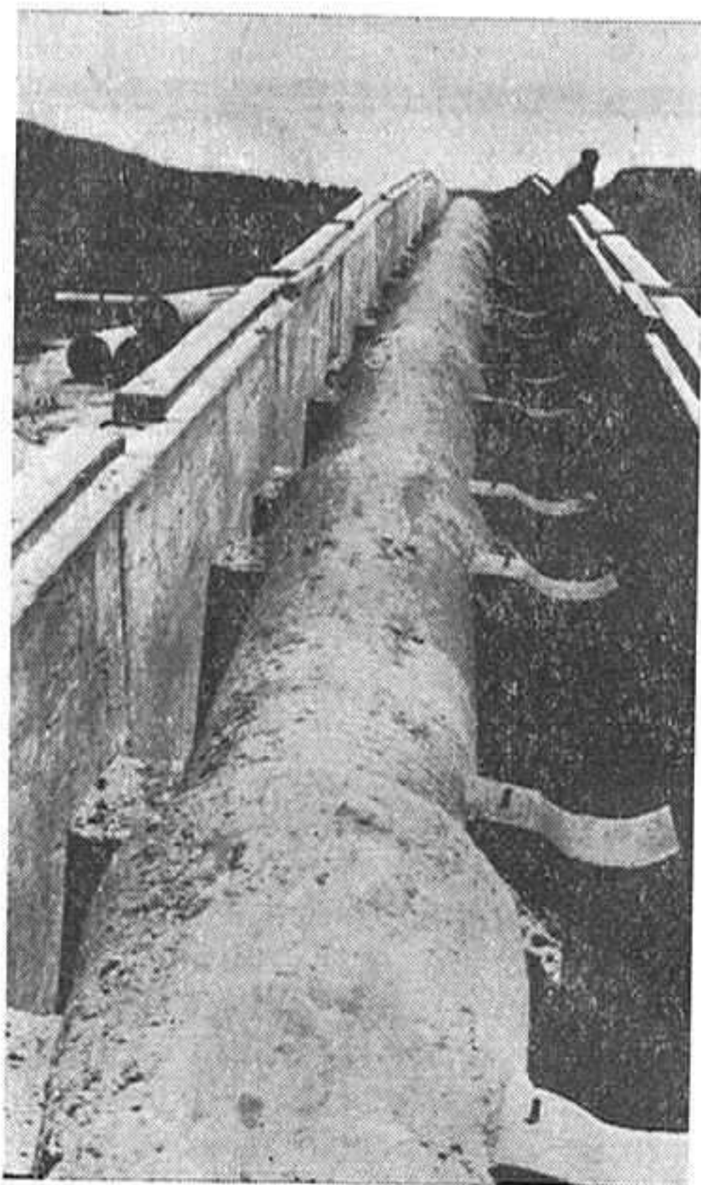
El caudal de agua potable del Sorbe llega a nuestra ciudad por esta tubería, que ya ha cruzado el río Henares. La figura del hombre que aparece en la parte superior da idea del diámetro de estos tubos.
