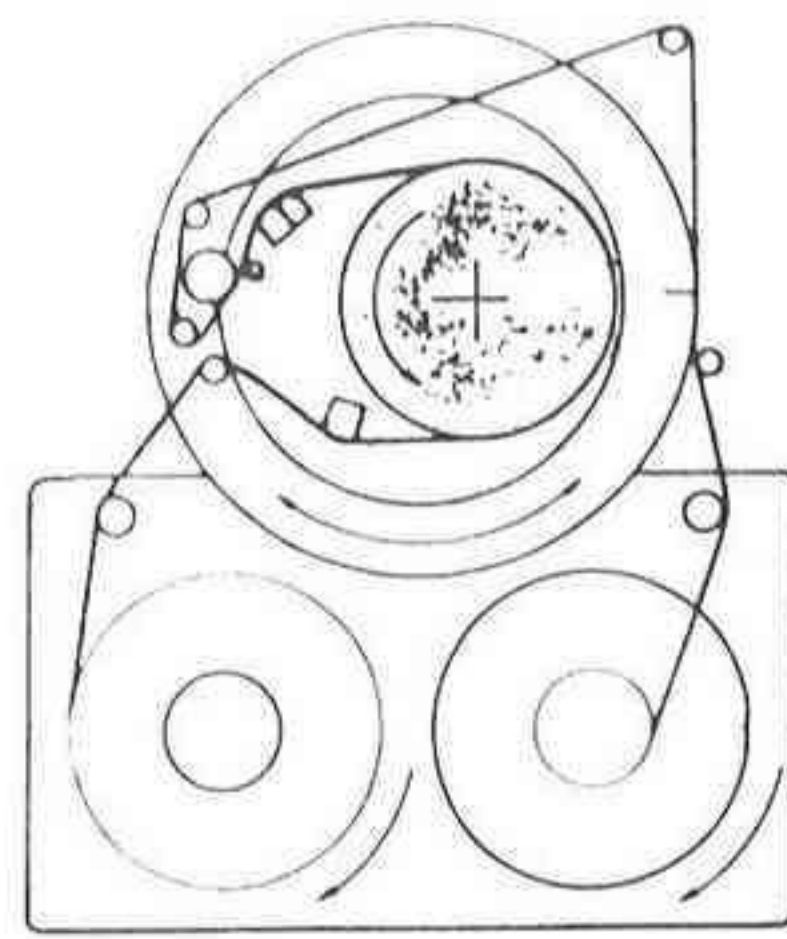
Sistema de carga en U de Grundig y en M de Philips
