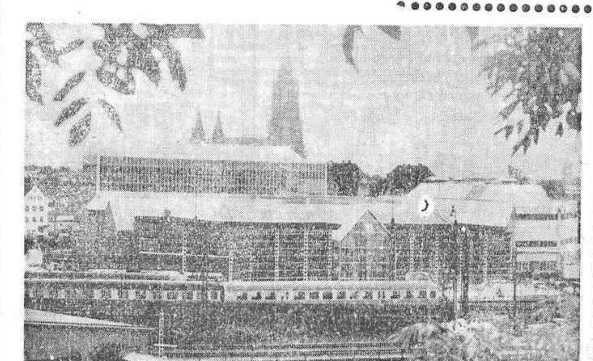
ULM. — No lejos de la catedral de Ulm (RFA), cuya silueta se ve al fondo, acaba de inaugurarse la compañía municipal de electricidad su nuevo edificio de oficinas, al que se ha dotado de doble fachada de cristal. La segunda fachada se halla a un metro de distancia de la otra. Con ello se consigue el aislamiento del edificio y se ahorra energía, aparte de que en los días soleados de invierno se aprovecha la energía térmica del sol. La compañía de electricidad de la ciudad danubiana de Ulm da el ejemplo a la hora de ahorrar energía. — (Foto: Dag-BERND KRUG)
