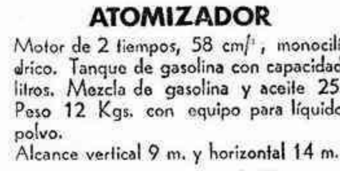
ATOMIZADOR
