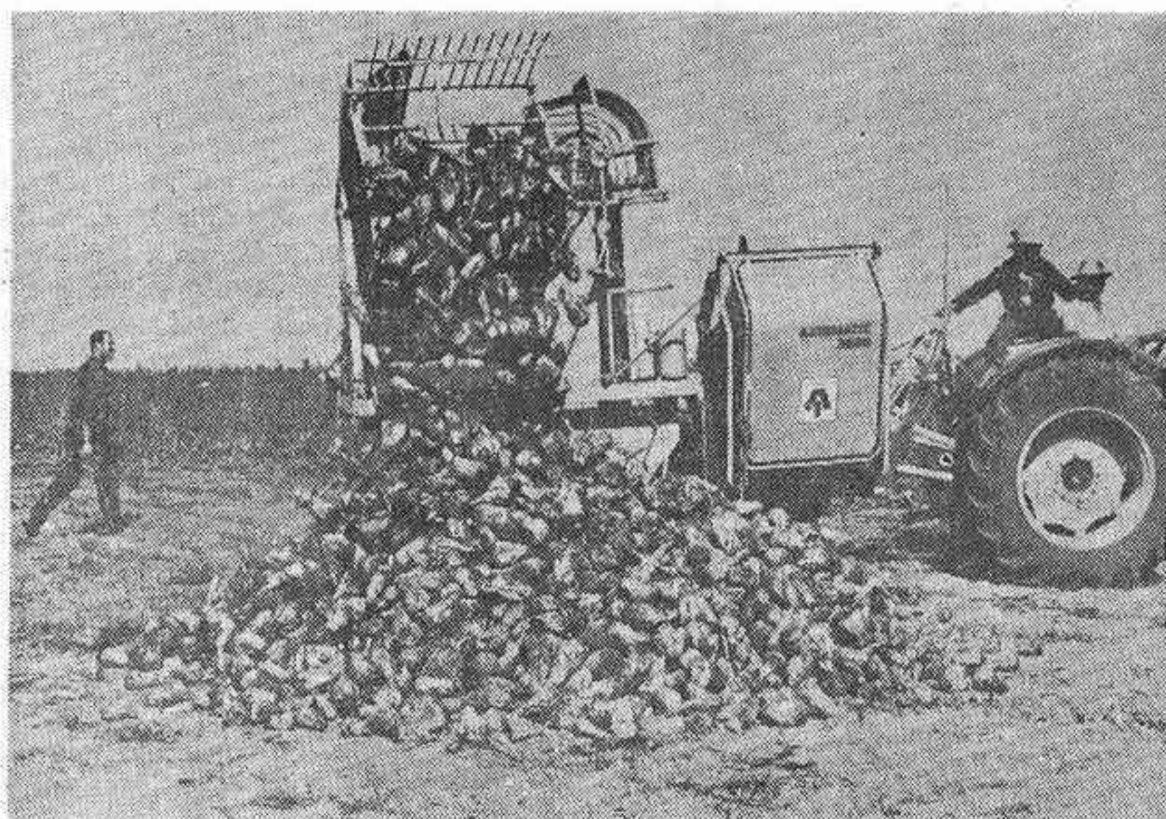
LEBRJA (Sevilla).— Una de las maquinarias que participaron en la X Demostración Internacional de Recolección Mecanizada de Remolacha, durante su trabajo ante numerosos agricultores de esta región. Concurrieron máquinas españolas, alemanas, checoslovacas, francesas e italianas. La demostración se realizó en la Hacienda Micones y estuvo organizada por la Dirección General de la Producción Agraria. — (Telefoto Cifra Gráfica)
