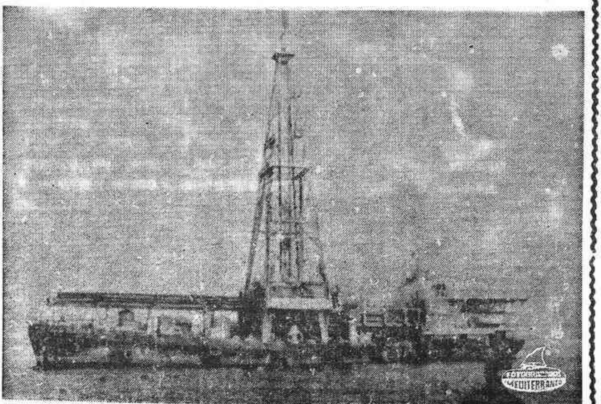
SAN CARLOS DE LA RAPITA. — Vista general del barco perforador «Giomar IV» situado a 22 kms. de la costa, donde se están llevando a cabo prospecciones petrolíferas. — (Telefoto CIFRA)
