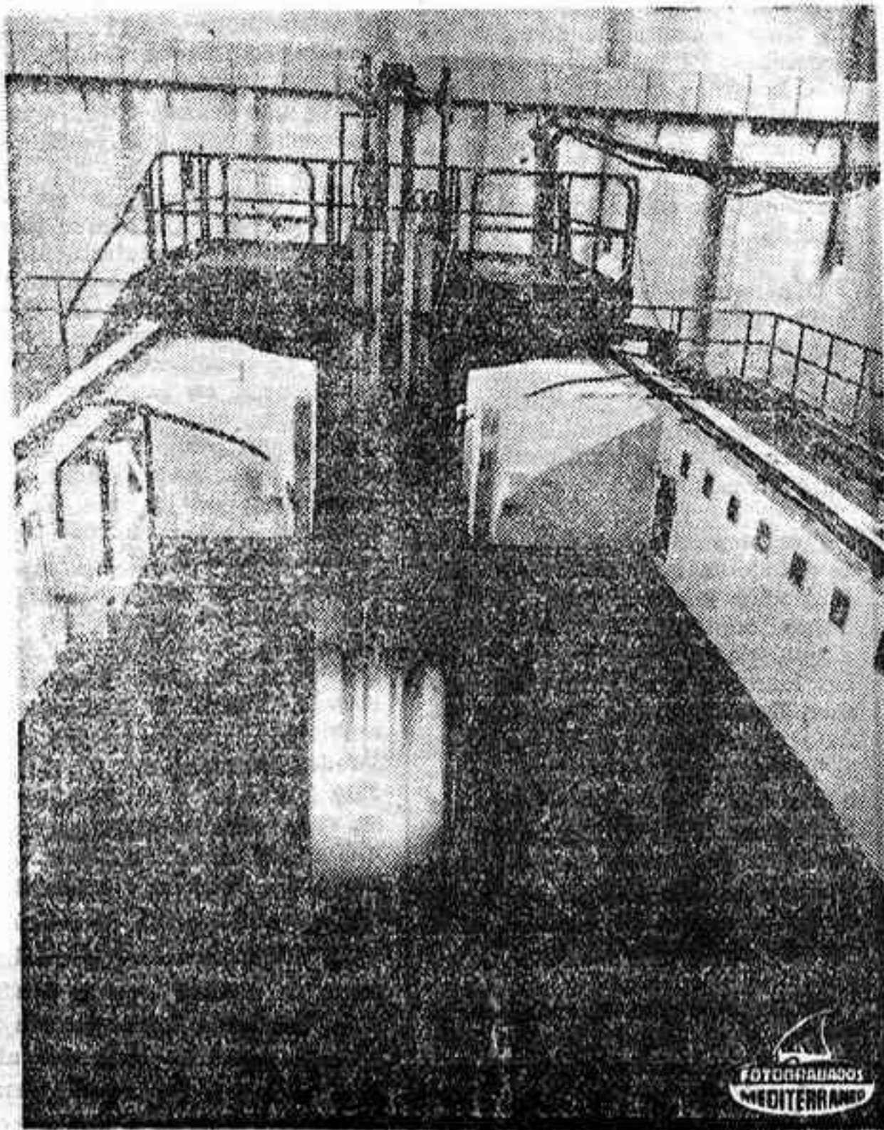
Vista del núcleo del reactor J. E. N. 1. — (Foto Pyresa).
