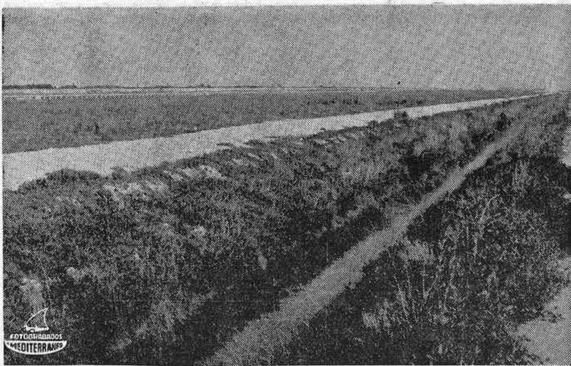
COLECTOR PRINCIPAL DE UNA DE DRENAJE. EN EL ANGULO SUPERIOR DERECHO ESTA LA ESTACION DE BOMBEO
