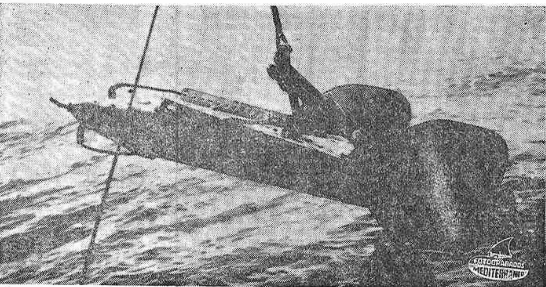
Prototipo de divergente realizado por el Instituto de Investigaciones Pesqueras, para análisis en continuo del mar, a bordo del buque oceanográfico italiano Bannock
