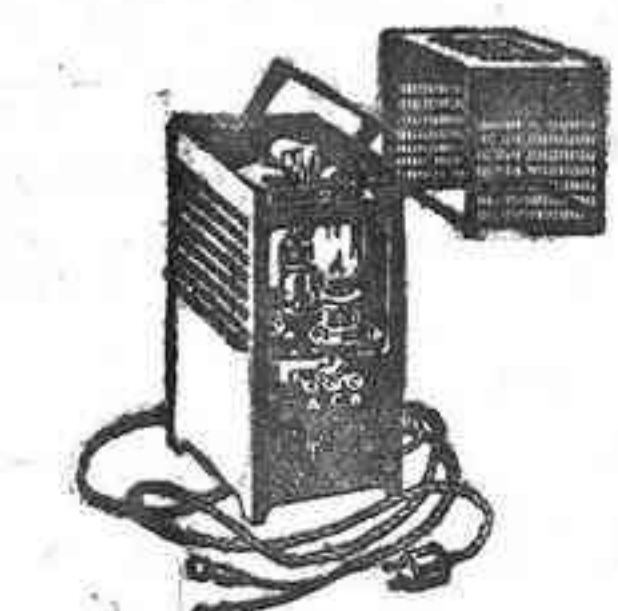
Rectificador Philips para garage Seguro — Práctico — Económico
