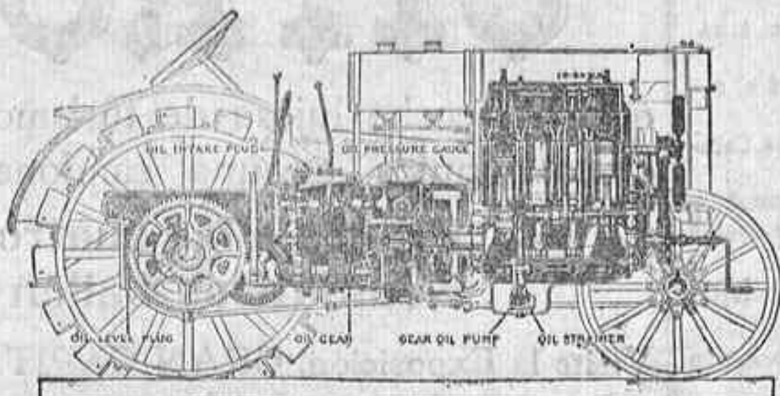
Tractor DEERING nuevo modelo.
