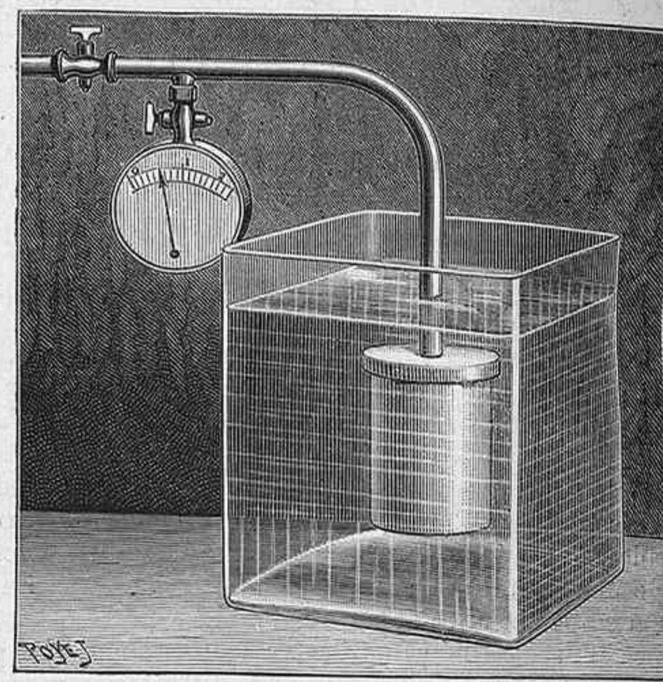
Fig. 2. Dispositivo para el estudio de la reacción capilar en las membranas ó vasos porosos.
