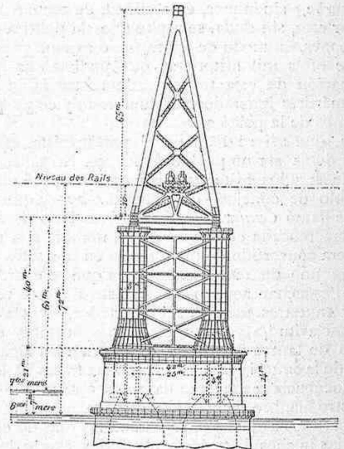
Fig. 2.—Sección transversal en una pila
