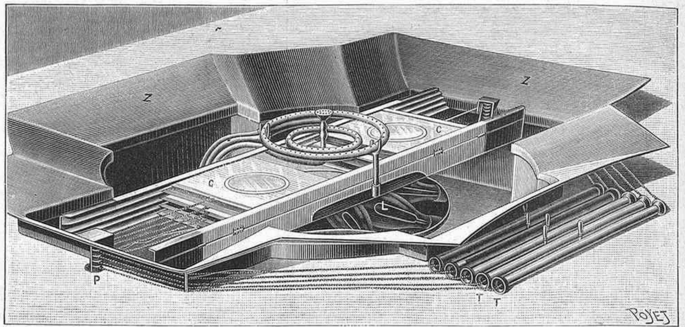
Fig. 2.—Mecanismo de la fuente luminosa de M. Gaston Menier
