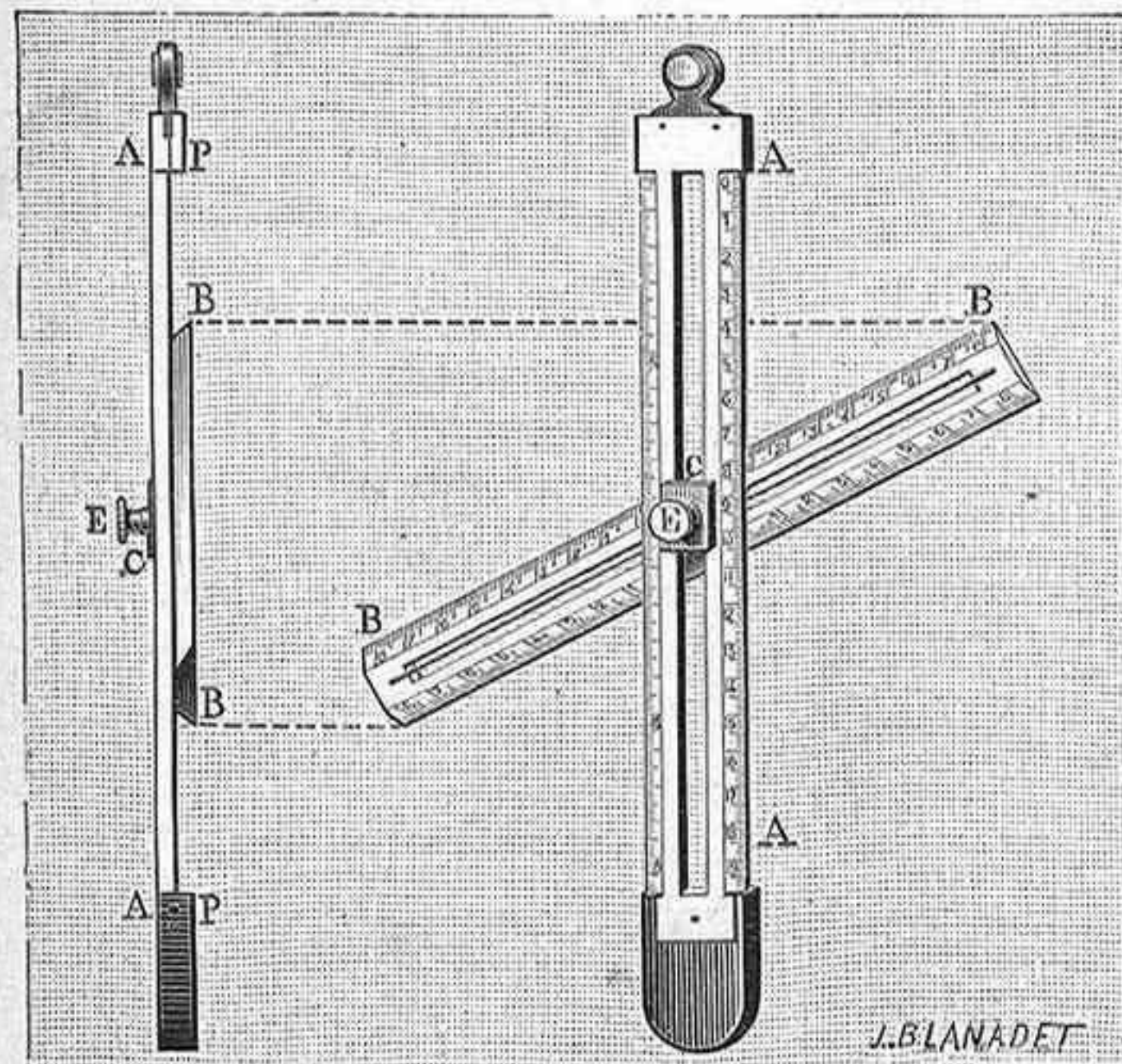
Fig. 3. - El similígrafo-nivel
