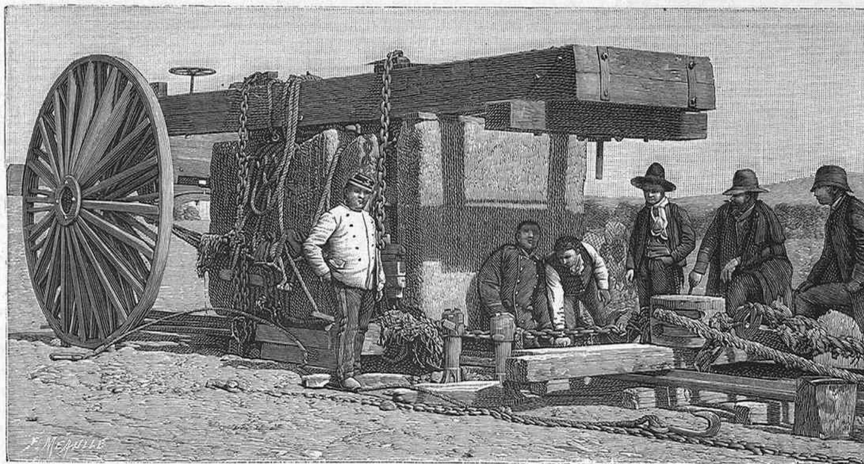
Fig. 2. - El monumento de la Diosa del agua colocado en el carro de transporte
