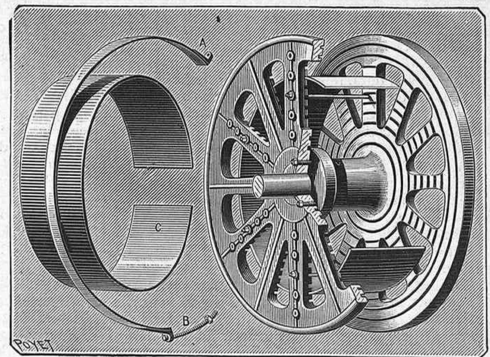
Polea de diámetros variables
