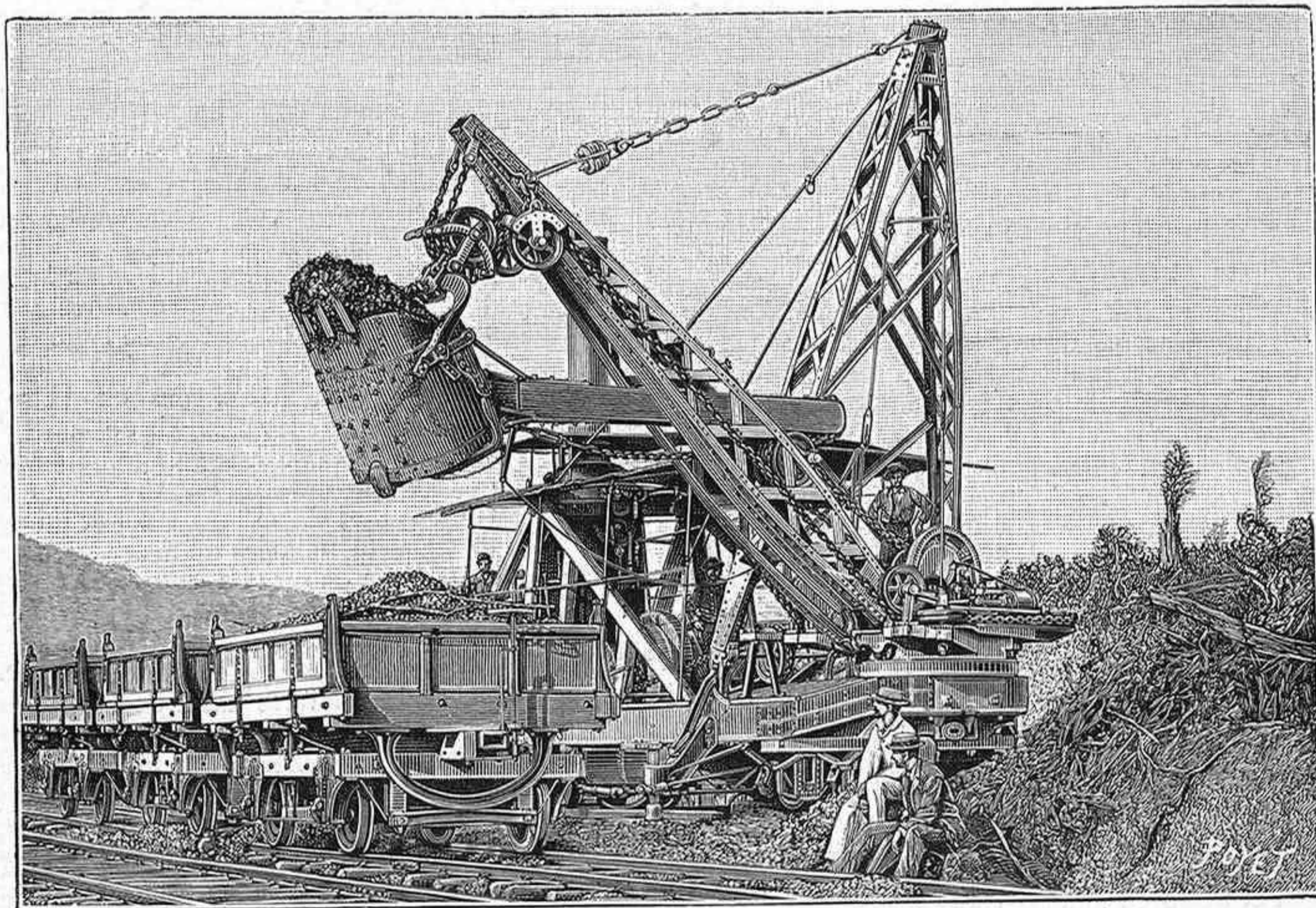
Trabajos de perforación del istmo de Panamá. - El excavador Osgood en la zanja grande La Culebra
