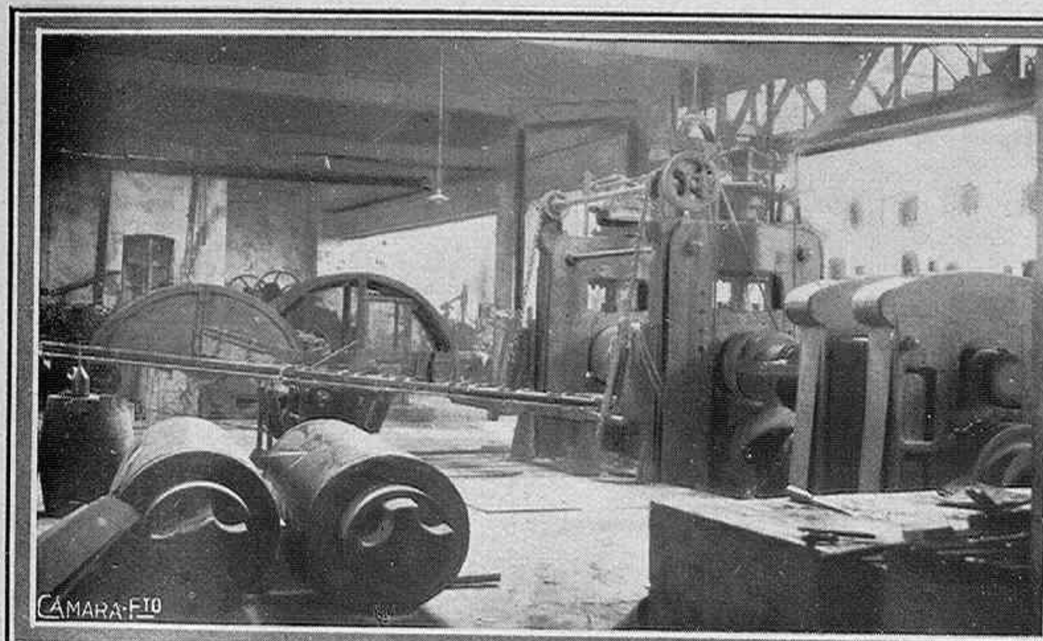
Sala de los grandes cilindros de laminar
