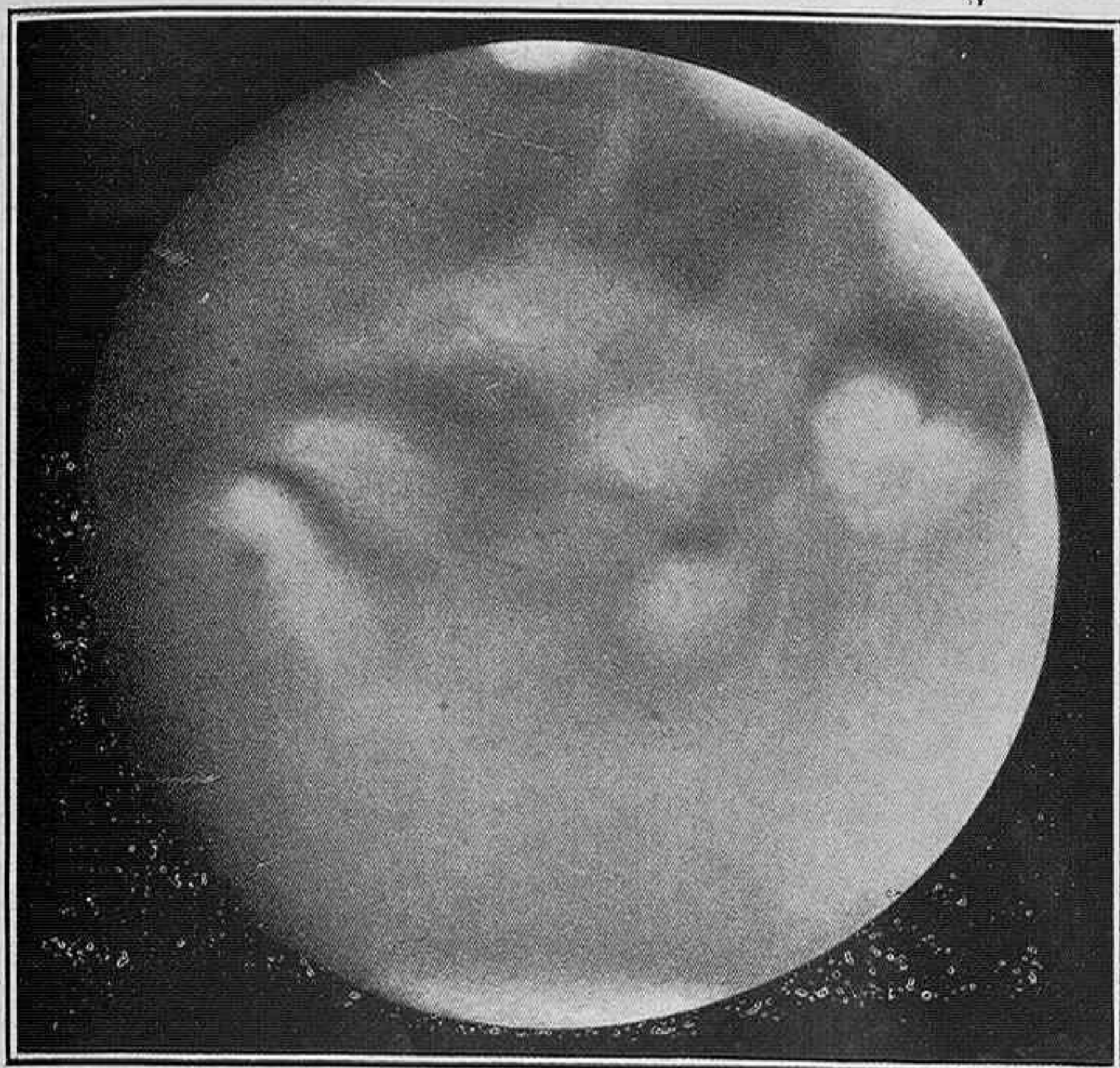
Aspecto de Marte el día 30 de Septiembre último, según las observaciones efectuadas en Meudón por el astrónomo Antoniadi
