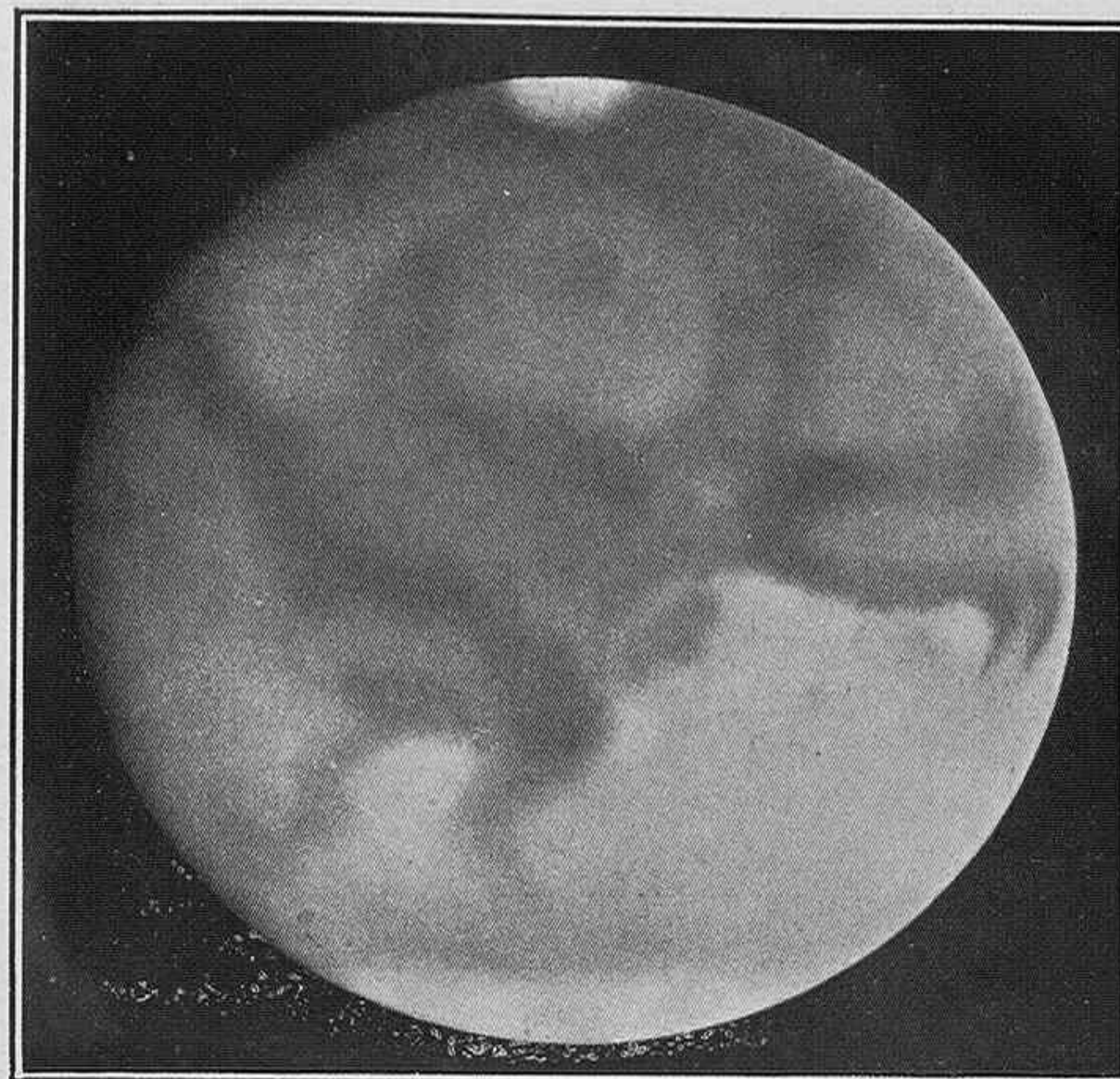
Notables cambios efectuados en el aspecto de Marte, y que han sido advertidos el 18 de Octubre, durante las observaciones hechas por el astrónomo Antoniadi en Meudón
