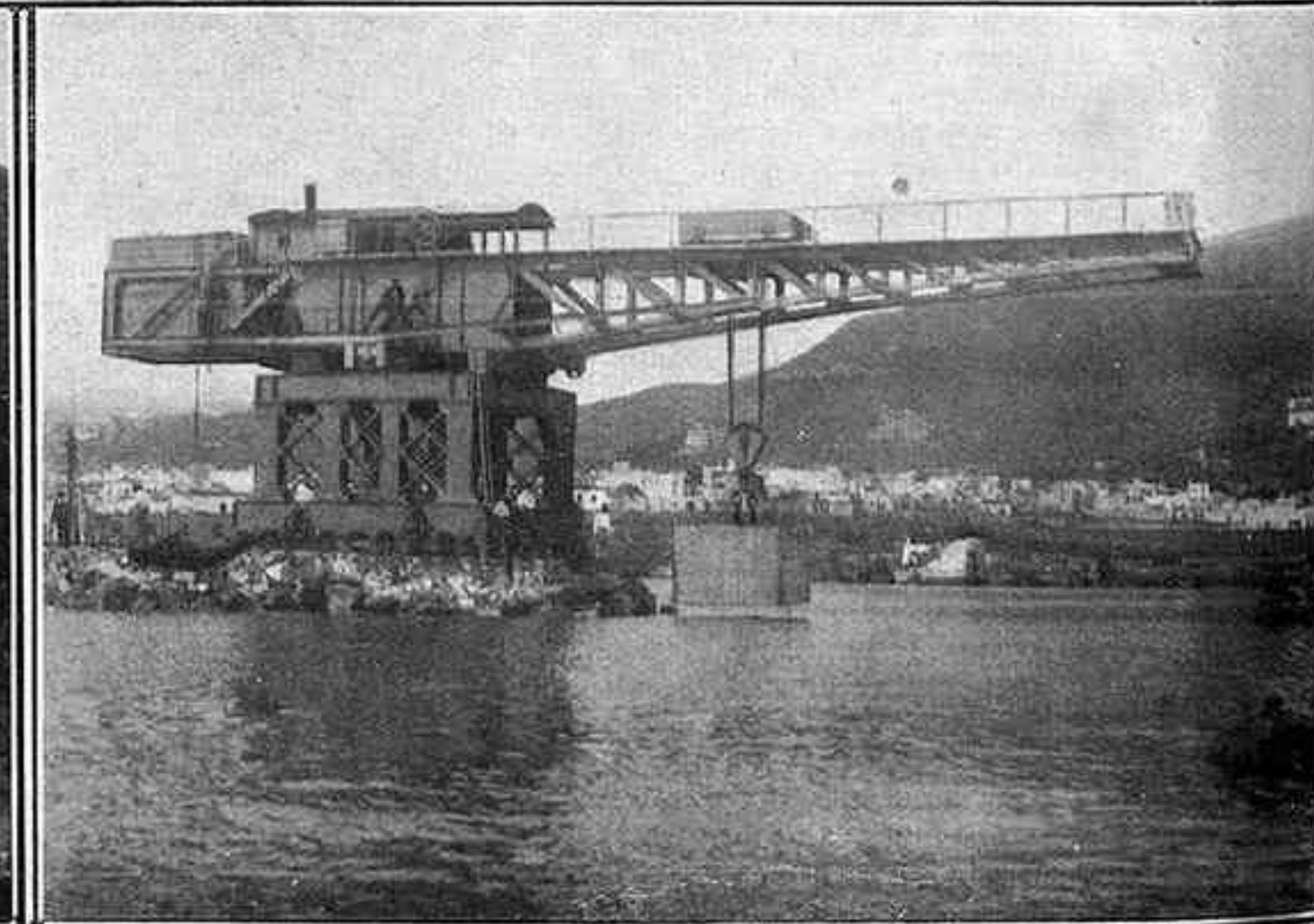
La grúa "Titán" colocando un bloque de cuarenta y cinco toneladas en las obras del puerto
