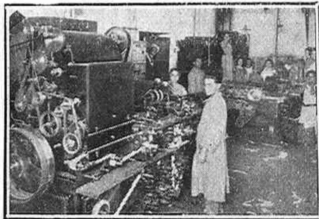
Salón de máquinas de la Fábrica de Tabacos «La Belleza»
