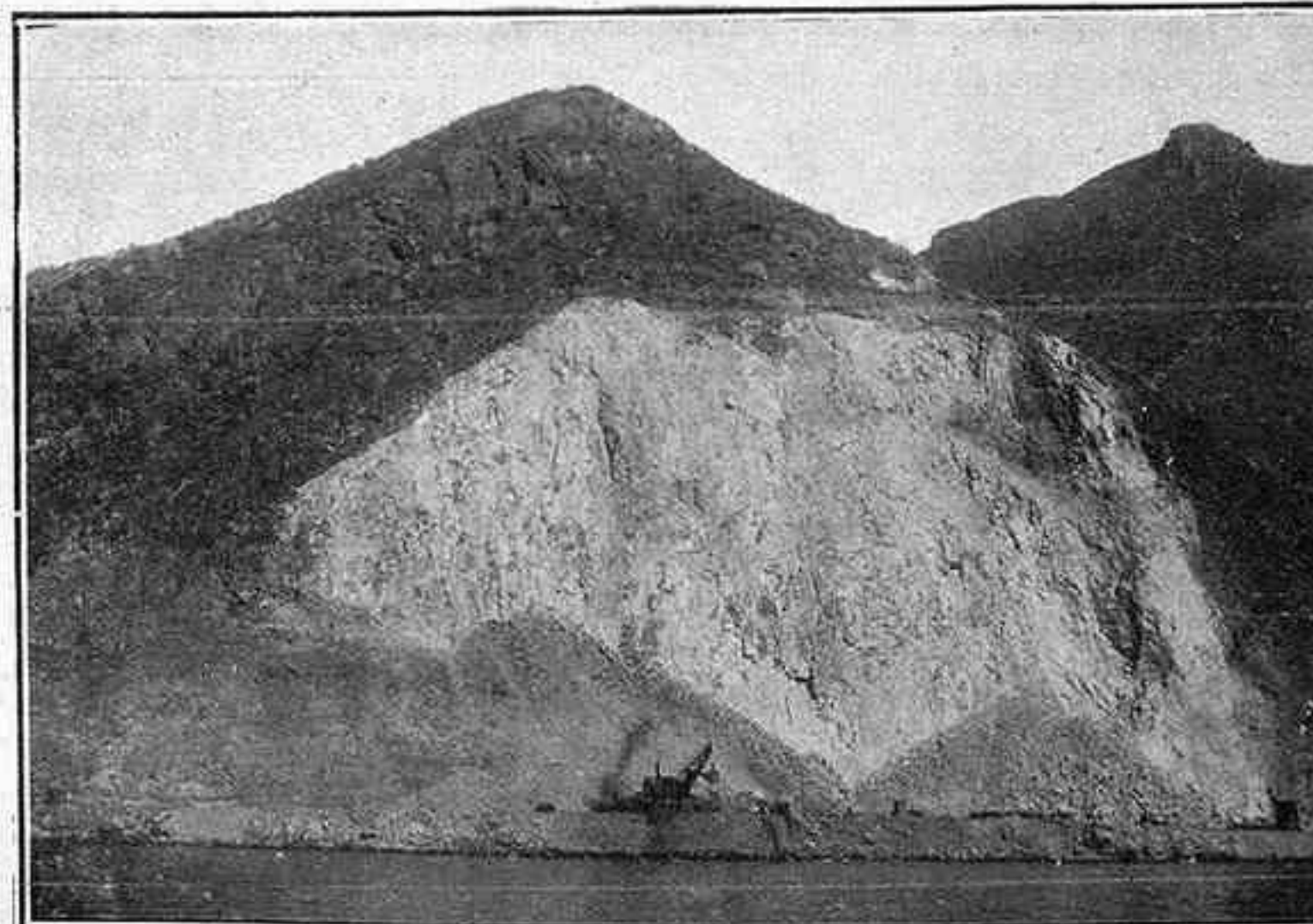
Cantera "La Jurada", de donde se extrae la piedra para la escollera del dique
