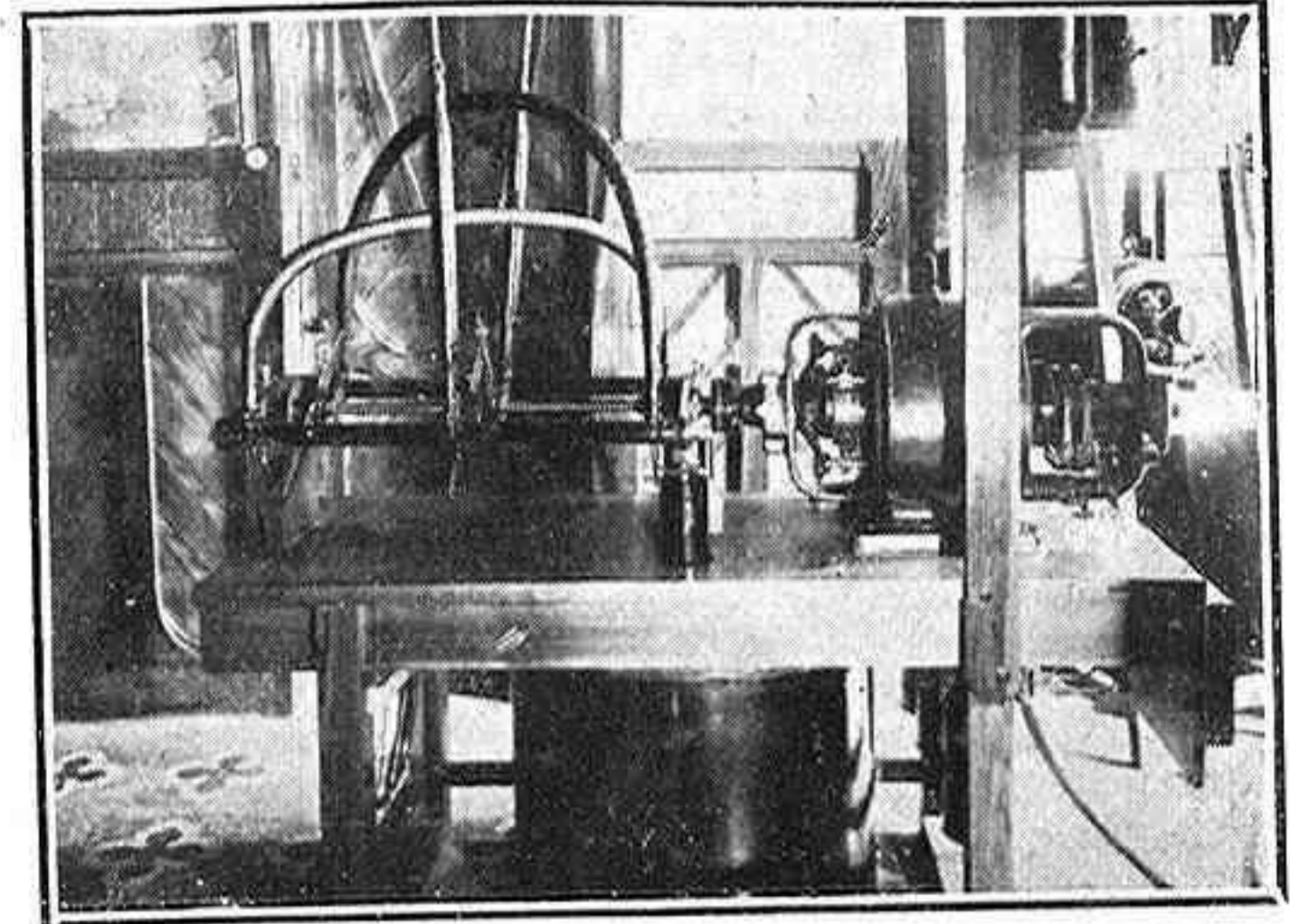
Contacto giratorio de Siemens para radioscopia y radiografía
