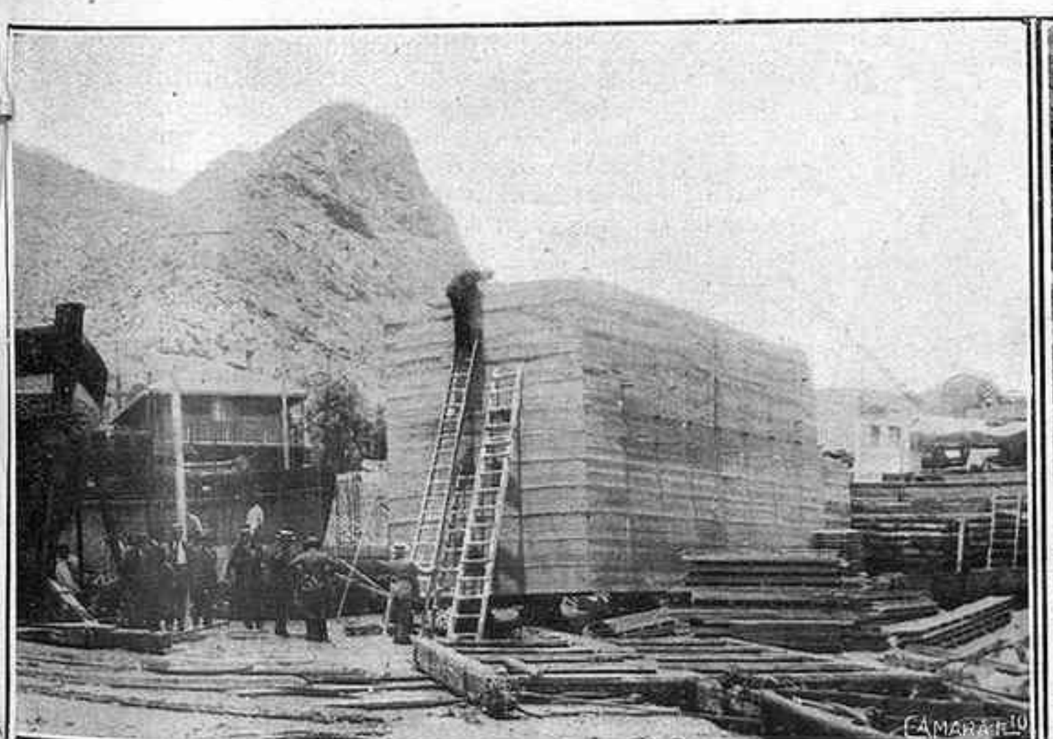
Cajón de hormigón armado construido en el astillero de la Junta para la Avenida Marítima
