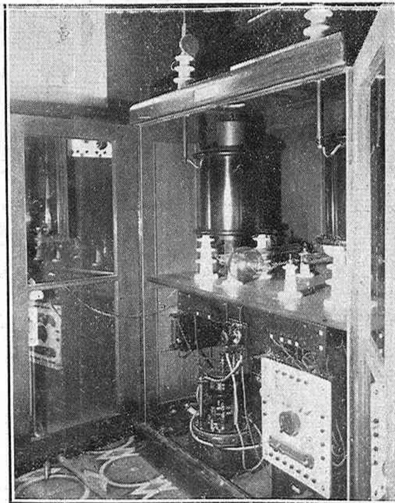
Aparato neosymmetrie de radioterapia profunda.
