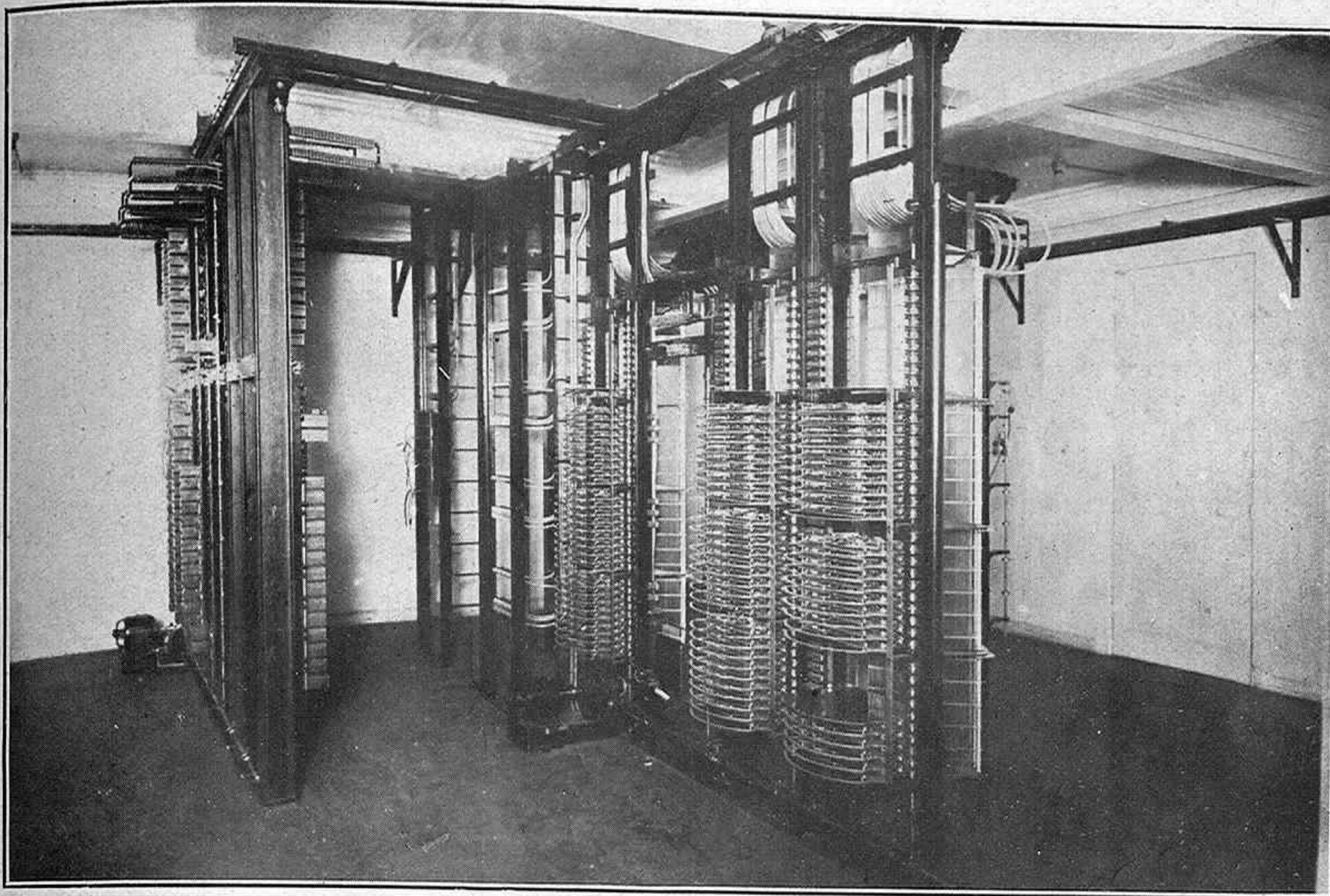
Central Provincial instalada en San Sebastián por la Excm. Diputación de Guipúzcoa
