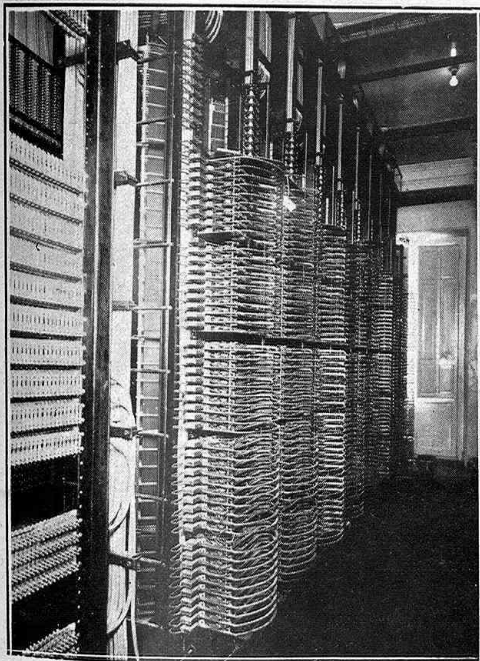
Vista parcial de uno de los bastidores de selectores de la Central Municipal de Teléfonos de San Sebastián
